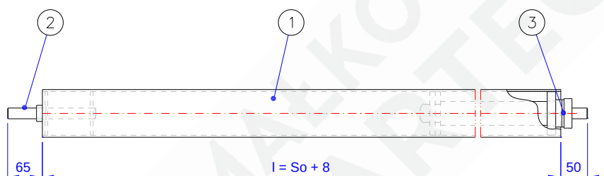
Rys. 6 – MARC-K(1)-01.03.00 [wał nawojowy]
