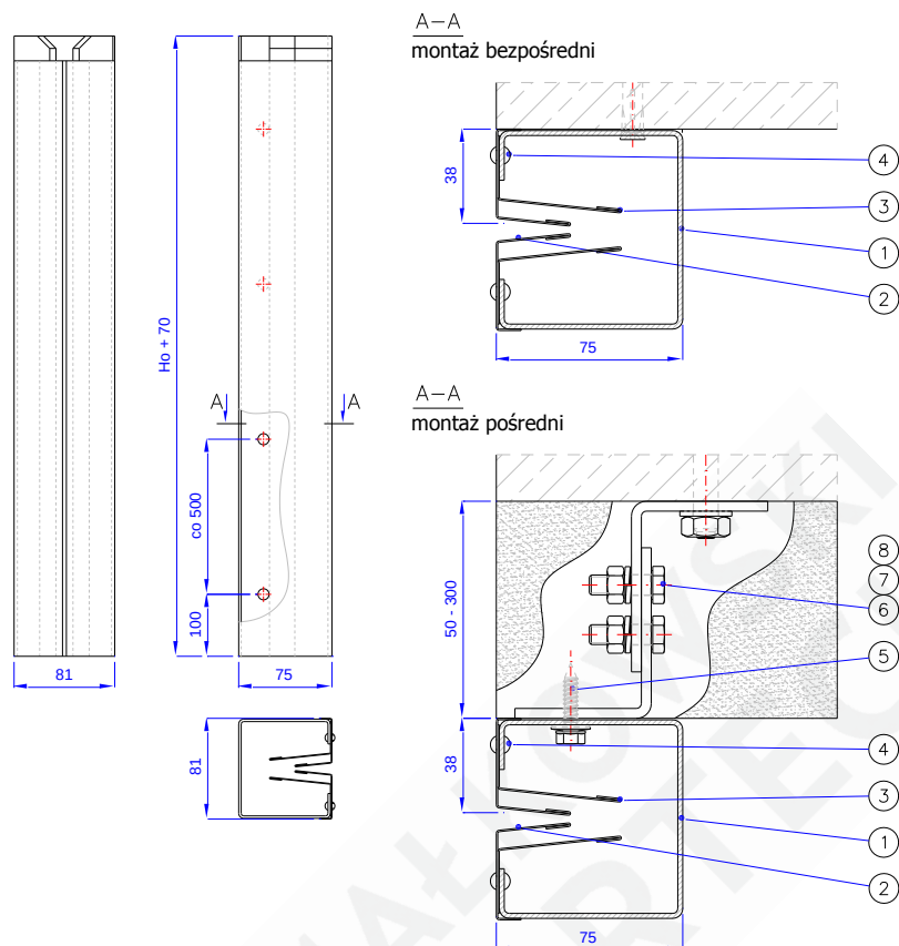
Rys. 5 – MARC-K(1)-01.02.00 [prowadnica]
