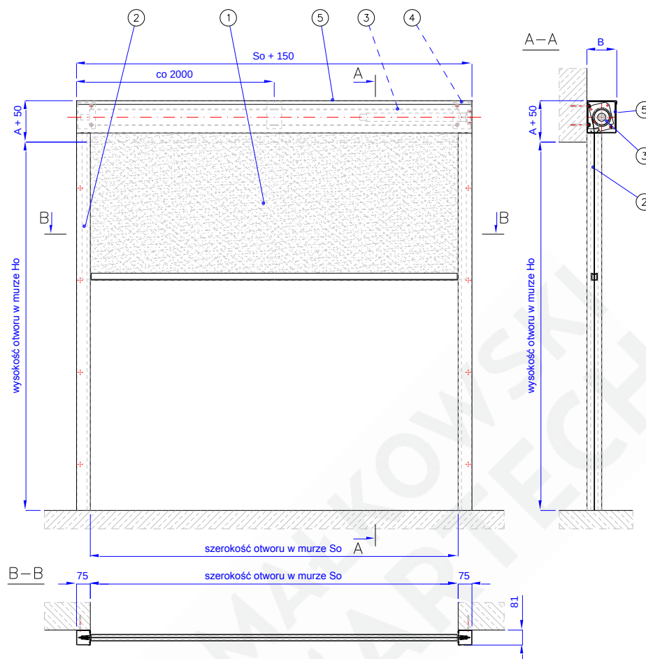
Rys. 1 – Przeciwpowozarowa brama kurtynowa typu MARC-K EW120/E120
