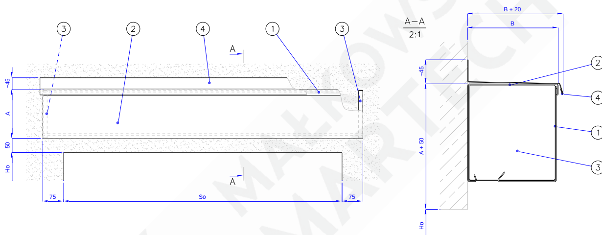
Rys. 8 – MARC-K(1)-01.05.00 [zespół osłon]
