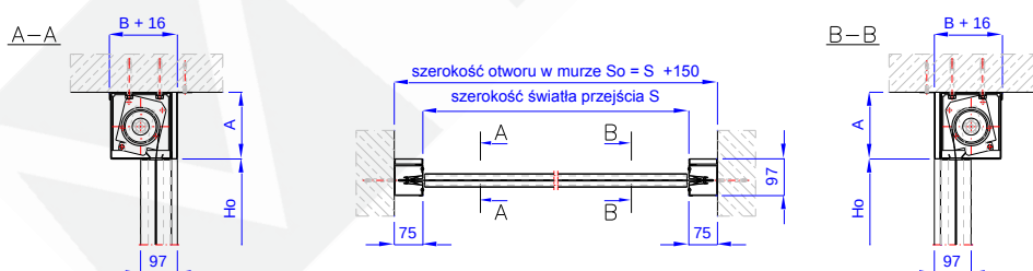
Rys. 2 – Przeciwpowozarowa brama kurtynowa typu MARC-K EW120/E120
