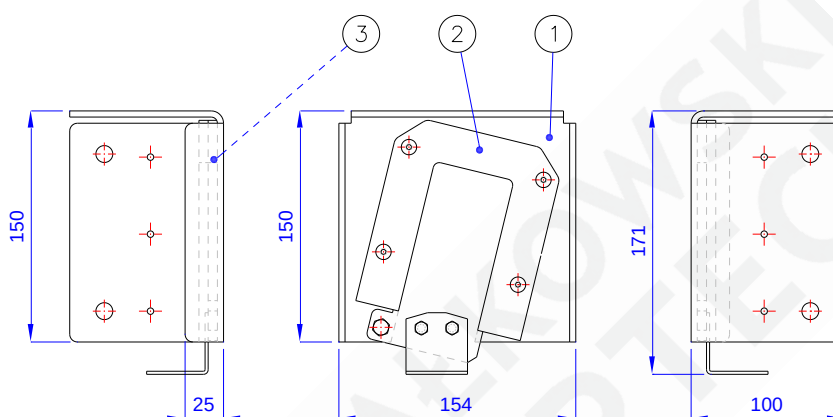
Rys. 7 – MARC-K(1)-01.04.00 [wspornik wału]
