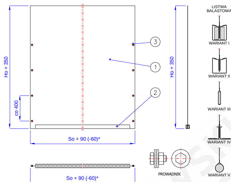
Rys. 4 – MARC-K(1)-01.01.00 [płaszcz bramy kurtynowej]
