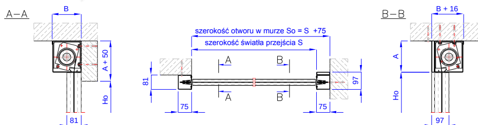
Rys. 3 – Przeciwpowozarowa brama kurtynowa typu MARC-K EW120/E120
