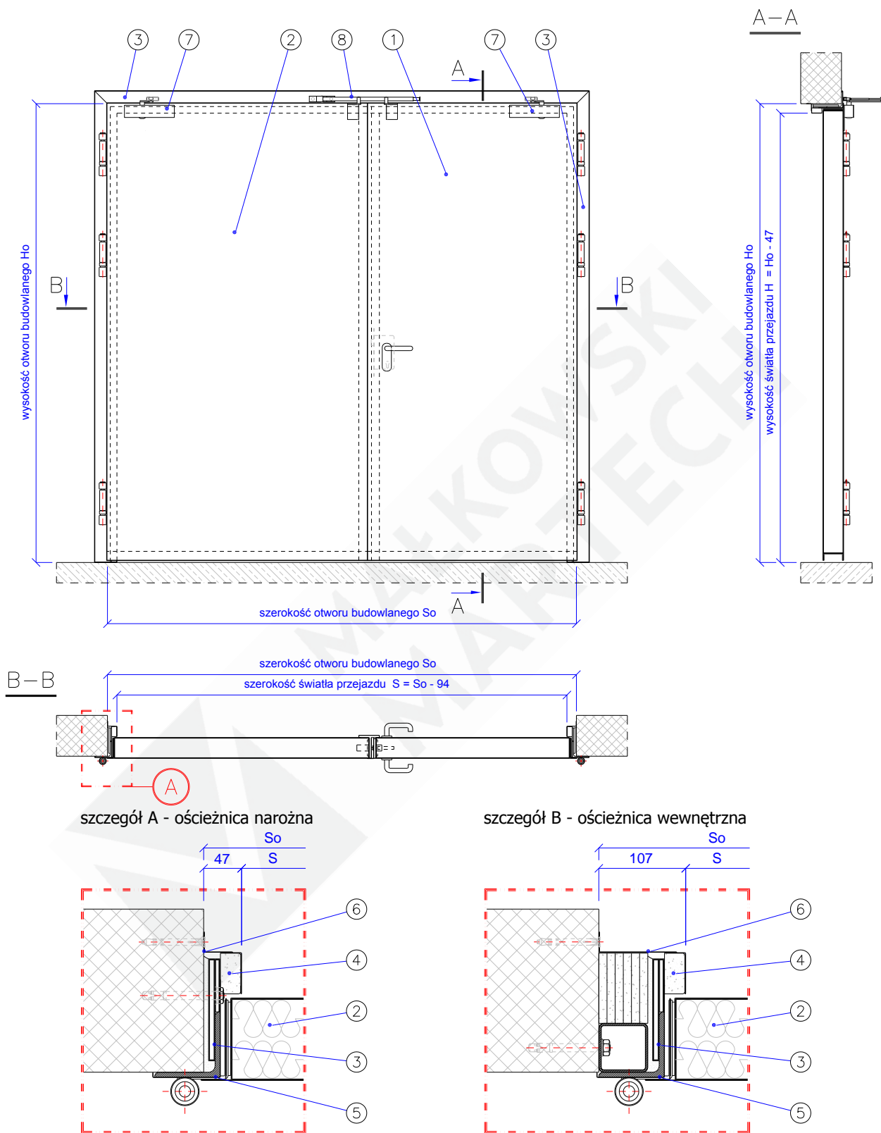
Rys. 1 – Przeciwpowozarowa brama rozwierana typu MARC-D EI60
