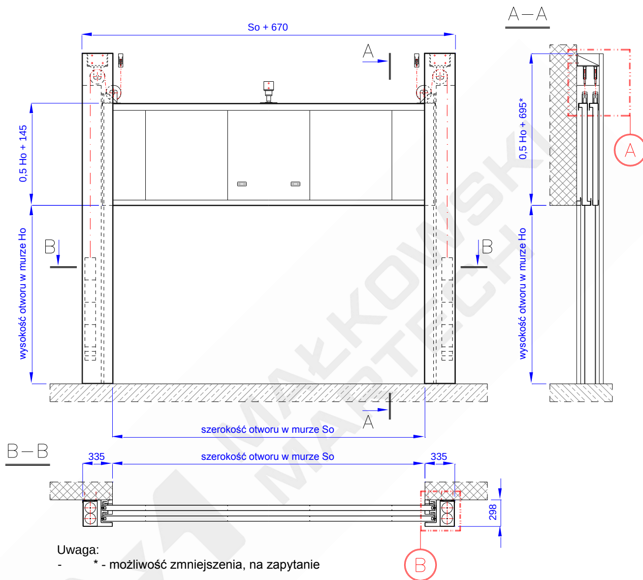
Rys. 1 – Przeciwpożarowa brama opuszczana, teleskopowa typu MARC-Ot EI60
