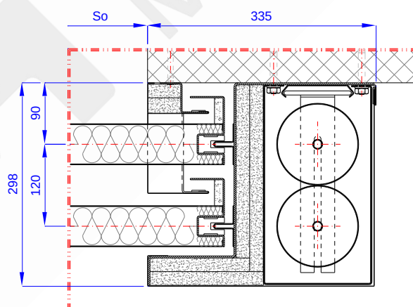
Rys. 3 – Szczegół B z Rys. 1
