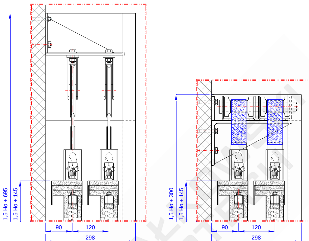
Rys. 2 – Szczegół A z Rys. 1 – w wariantcie z linami (z lewej strony) i pasami nośnymi (z prawej strony)
