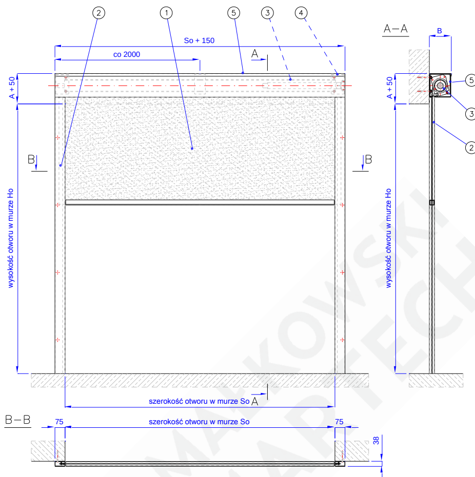
Rys. 1 – Przeciwpowozarowa brama kurtynowa typu MARC-K EW60/E90
