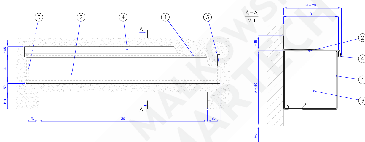
Rys. 8 – MARC-K(3)-01.05.00 [zespół osłon]
