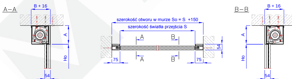
Rys. 2 – Przeciwpowozarowa brama kurtynowa typu MARC-K EW60/E90
