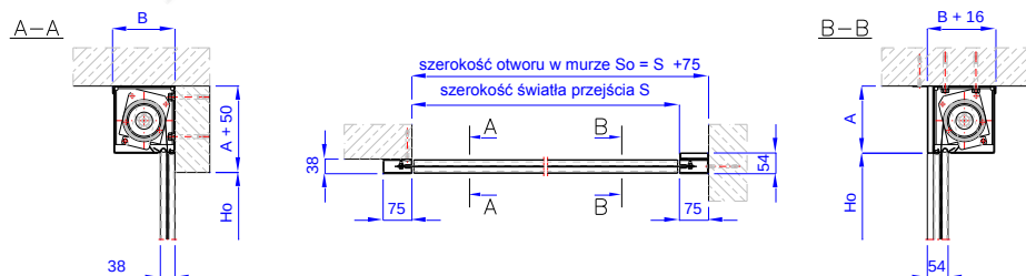
Rys. 3 – Przeciwpowozarowa brama kurtynowa typu MARC-K EW60/E90
