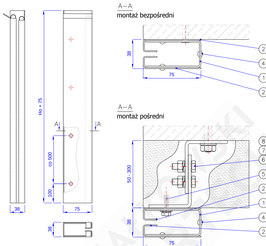
Rys. 5 – MARC-K(3)-01.02.00 [prowadnica]
