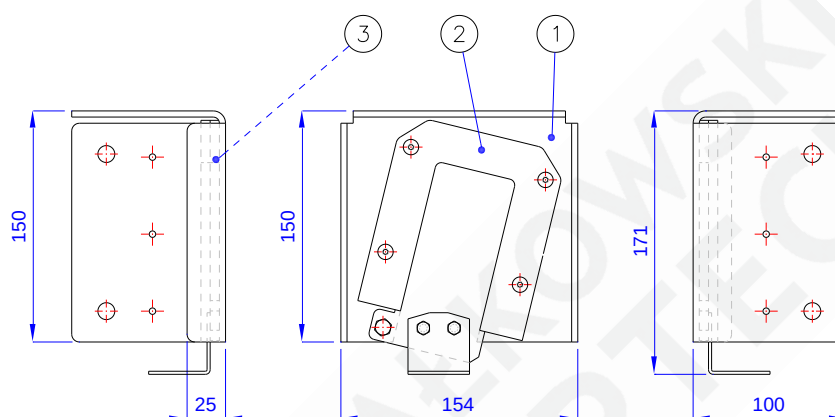
Rys. 7 – MARC-K(3)-01.04.00 [wspornik wału]
