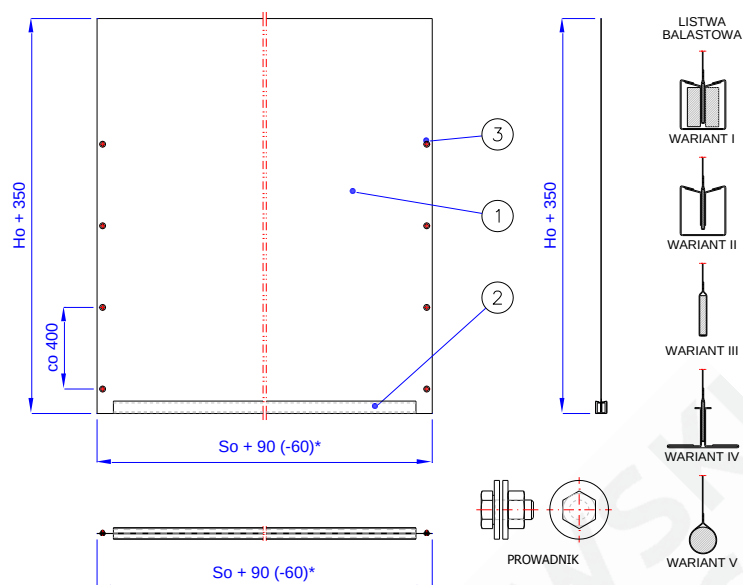
Rys. 4 – MARC-K(3)-01.01.00 [płaszcz bramy kurtynowej]
