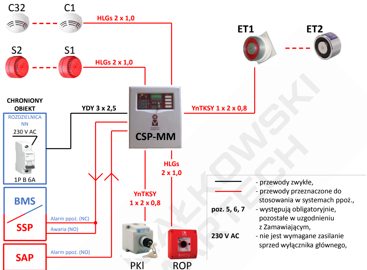
Schemat 1 – Układ sterowania MARC-Ot z trzymaczem elektromagnetycznym (zamykanie grawitacyjne)
