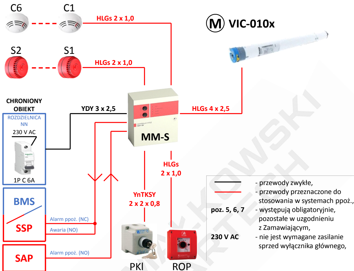
Schemat 3 – Układ sterowania MARC-Ot z napędem wewnętrznym (rurowym) 24 V DC
