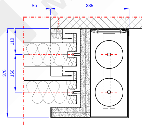
Rys. 3 – Szczegół B z Rys. 1
