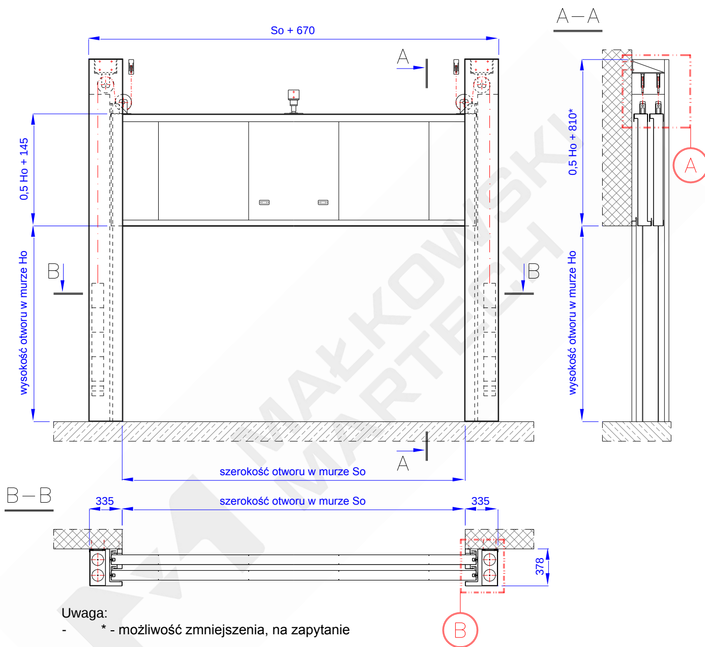
Rys. 1 – Przeciwpowozarowa brama opuszczana, teleskopowa typu MARC-Ot EI120
