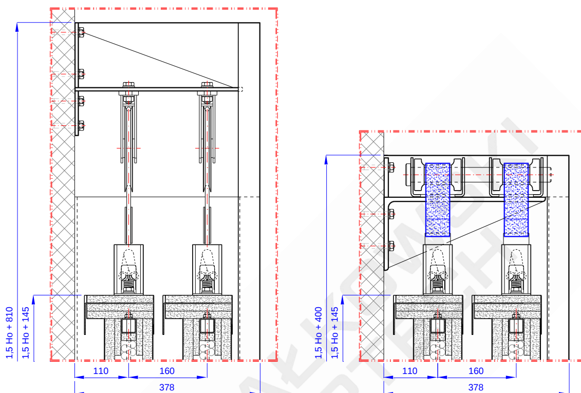
Rys. 2 – Szczegół A z Rys. 1 – w wariantcie z liniami (z lewej strony) i pasami nośnymi (z prawej strony)
