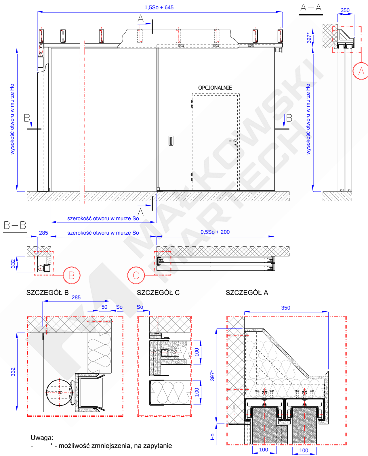
Rys. 1 – Przeciwpożarowa brama przesuwna, teleskopowa typu MARC-Pt EI120
