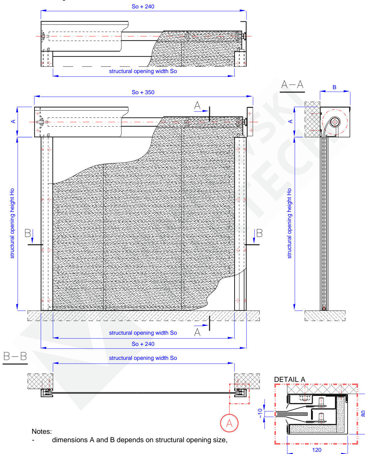
Fig. 1 – Fire protection curtain door MARC-Ok EI60
