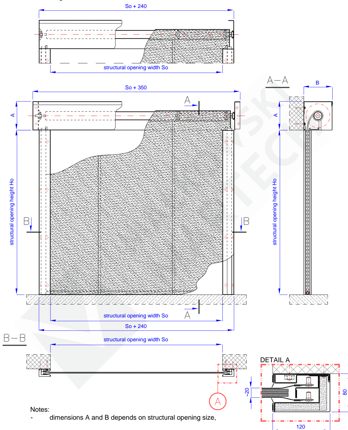
Fig. 1 – Fire protection curtain door MARC-Ok E190
