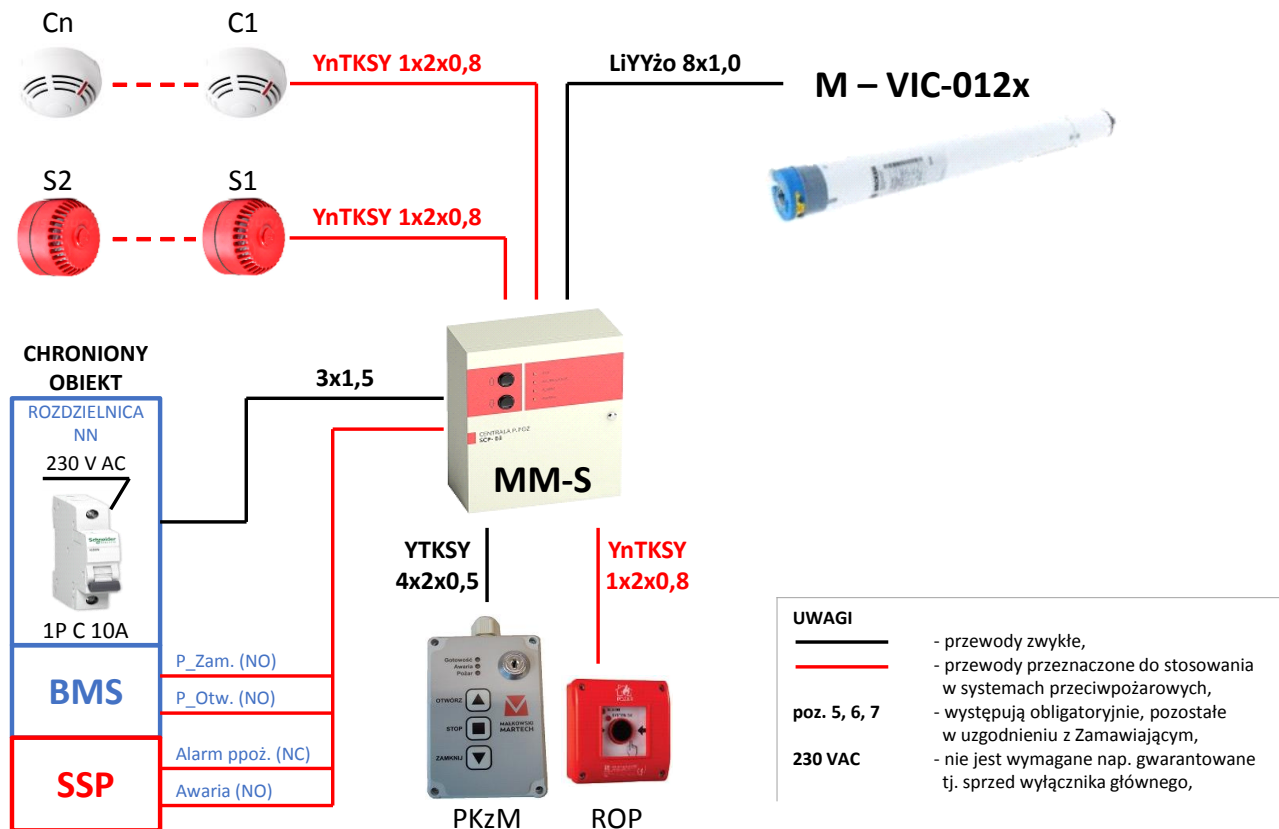
Rys. 12 – Zestaw osprzętu przeciwpożarowej bramy typu MARC-Ok z napędem VIC-012x
