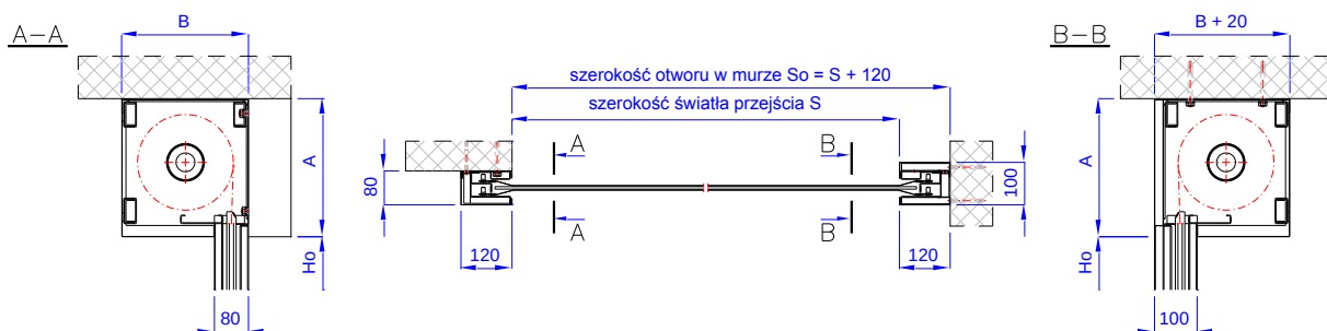
Rys. 4 - Przeciwpowozarowa brama kurtynowa typu MARC-Ok EI60 – zabudowa mieszana
