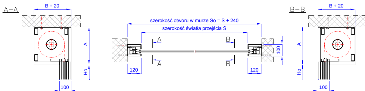
Rys. 3 - Przeciwpowozarowa brama kurtynowa typu MARC-Ok EI60 – zabudowa korytarzowa / wnąkowa (między równoległymi ścianami)
