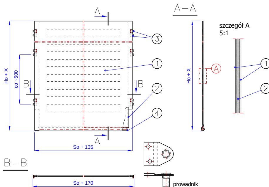
Rys. 6 - MARC-Ok60-01.01.00 [Płaszcz bramy]
