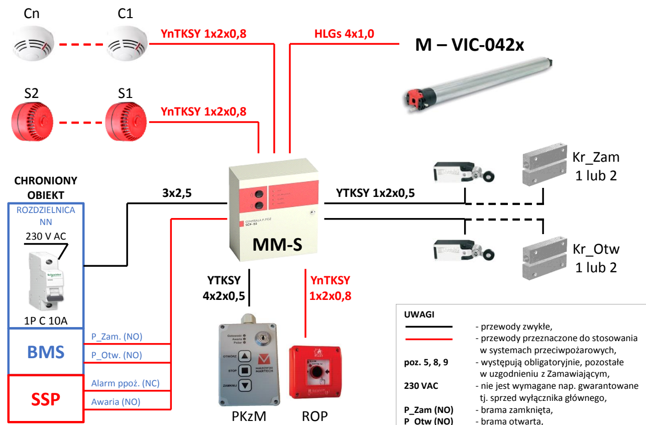
Rys. 14 – Zestaw osprzętu przeciwpożarowej bramy typu MARC-Ok z napędem VIC-042x z inwerterem
