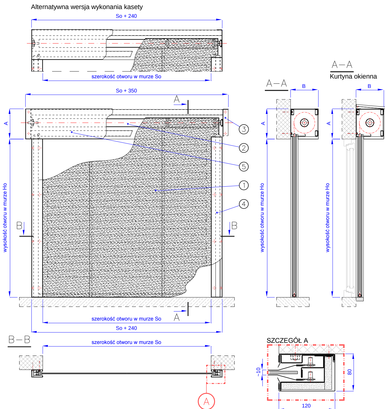
Rys. 2 - Przeciwpowozarowa brama kurtynowa typu MARC-Ok EI60
