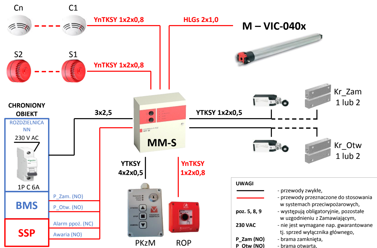
Rys. 11 – Zestaw osprzętu przeciwpożarowej bramy typu MARC-Ok z napędem VIC-0403
