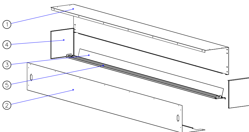
Rys. 10 - MARC-Ok60-01.05.00 [Zespół osłon]
