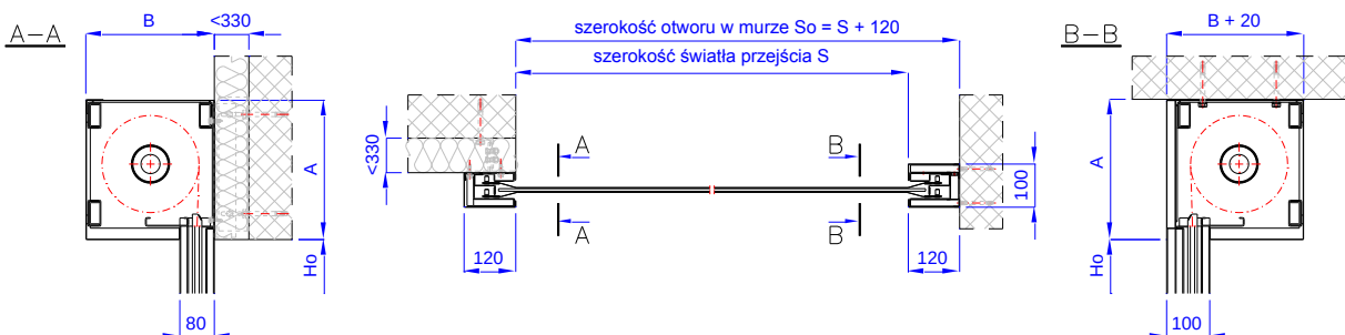
Rys. 5 – Przeciwpowozarowa brama kurtynowa typu MARC-Ok EI60 – zabudowa mieszana, jednostronnie na elementach dystansowych
