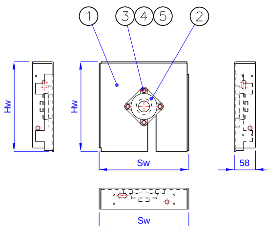
Rys. 8 - MARC-Ok60-01.03.00 [Wspornik wału]
