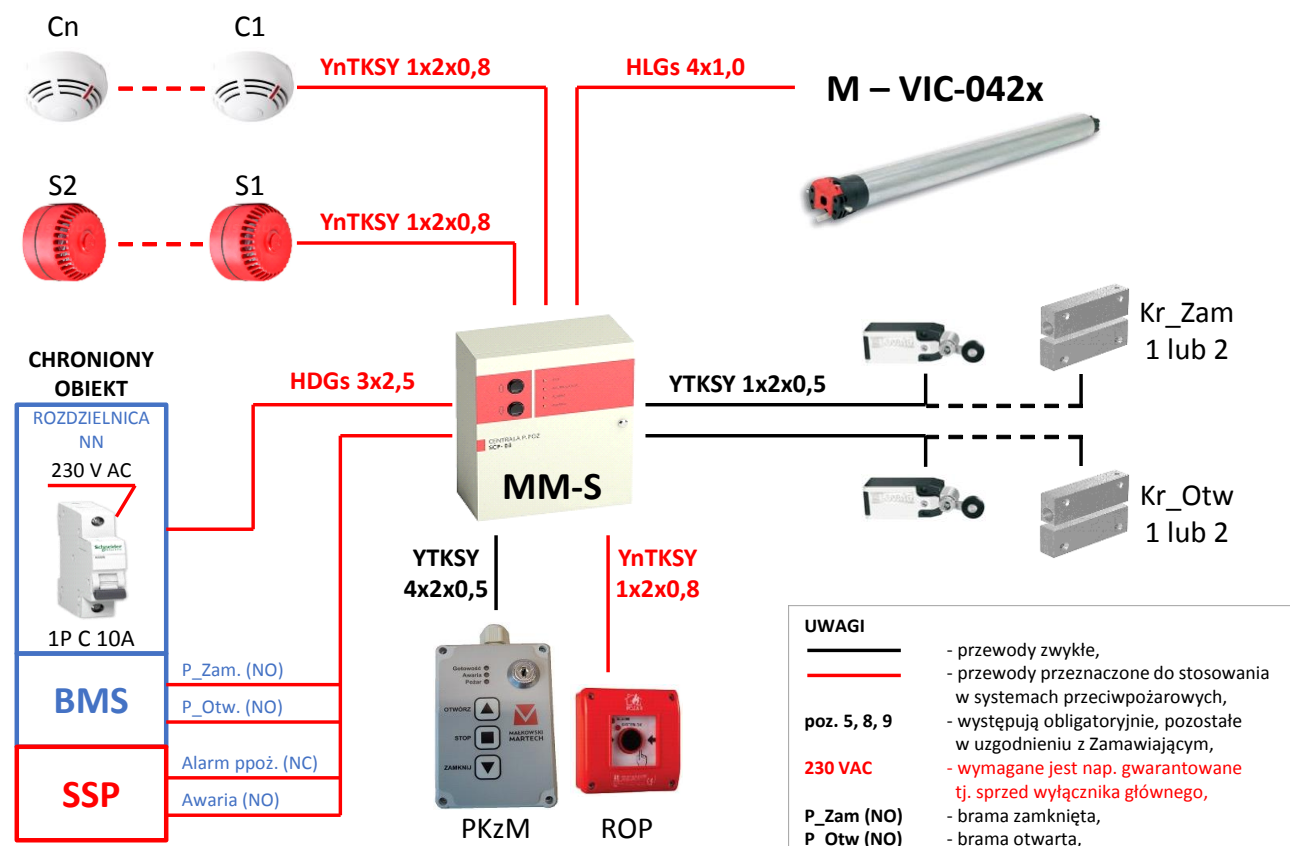
Rys. 13 – Zestaw osprzętu przeciwpożarowej bramy typu MARC-Ok z napędem VIC-042x
