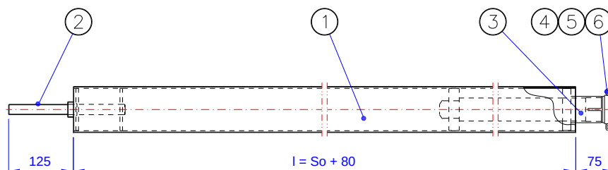
Rys. 7 - MARC-Ok60-01.02.00 [Wał nawojowy]
