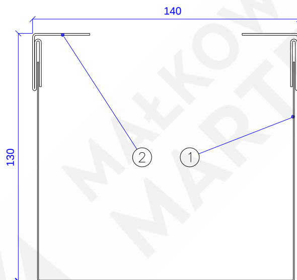
Rys. 11 – MARC-R60-01.10.00 [Osłona przeciwciężaru]
