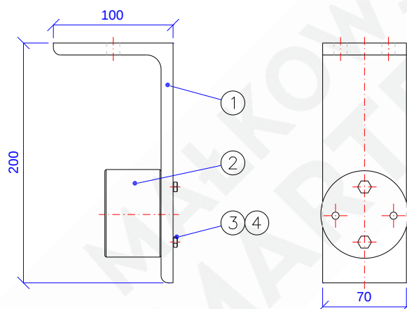
Rys. 8 – MARC-R60-01.07.00 [Zespół trzymacza elektromagnetycznego]
