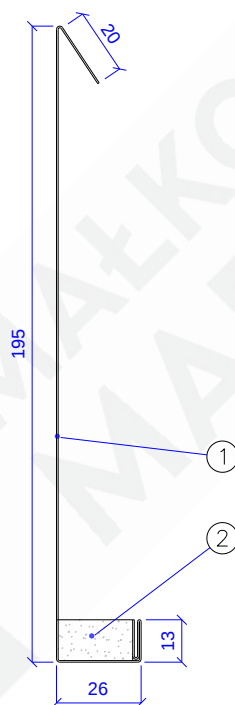
Rys. 10 – MARC-R60-01.09.00 [Osłona toru jezdnego]
