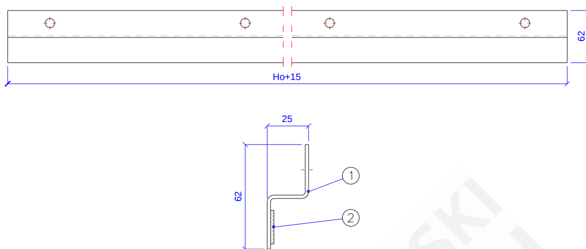
Rys. 5 – MARC-R60-01.04.00 [Przymyk naścienny]
