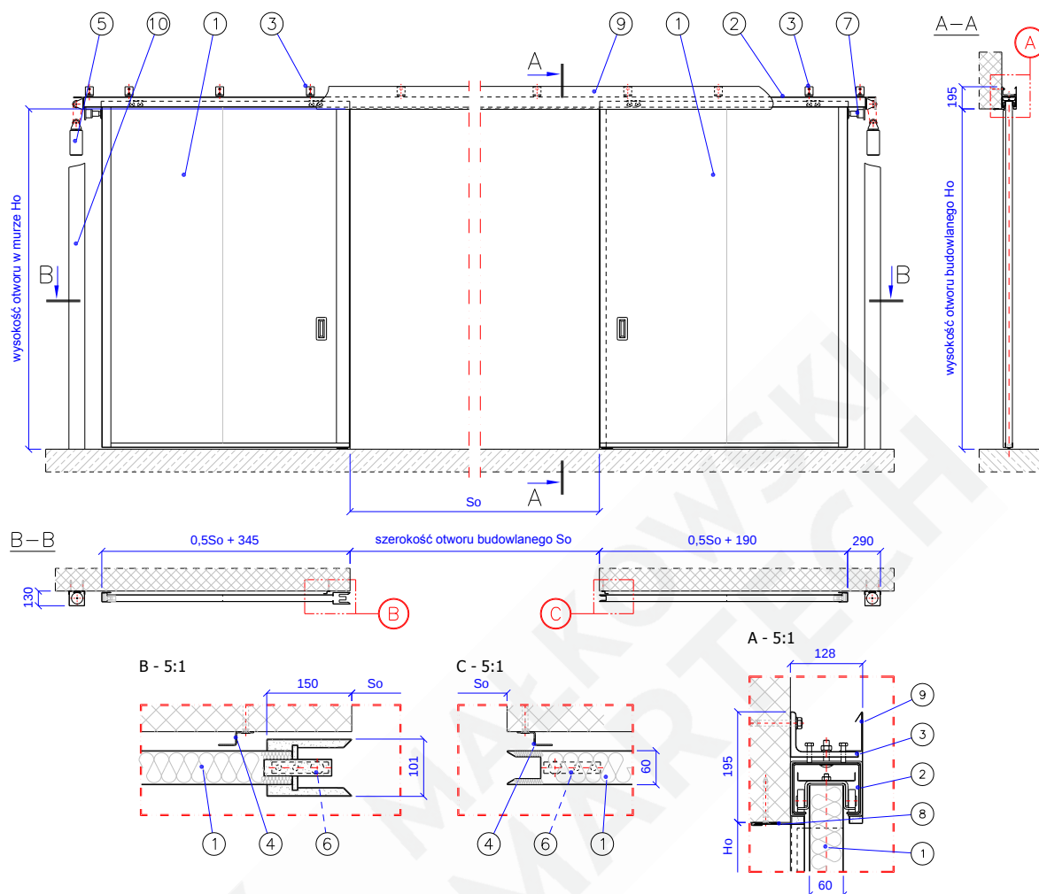
Rys. 1 – Przeciwpowozarowa brama rozsuwana typu MARC-R EI60
