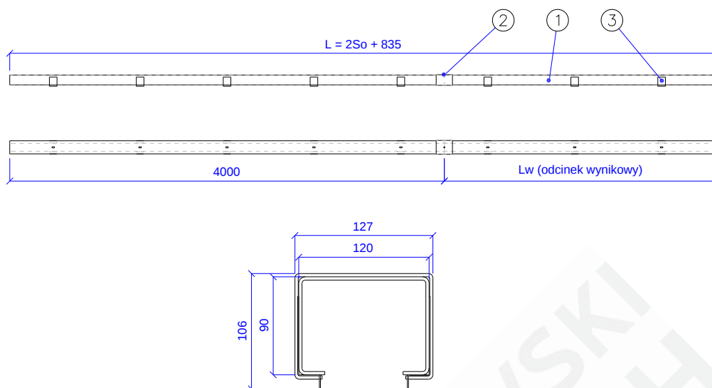
Rys. 3 – MARC-R60-01.02.00 [Tor jezdny]
