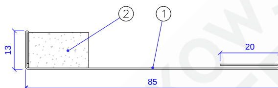
Rys. 9 – MARC-R60-01.08.00 [Osłona nadproża]
