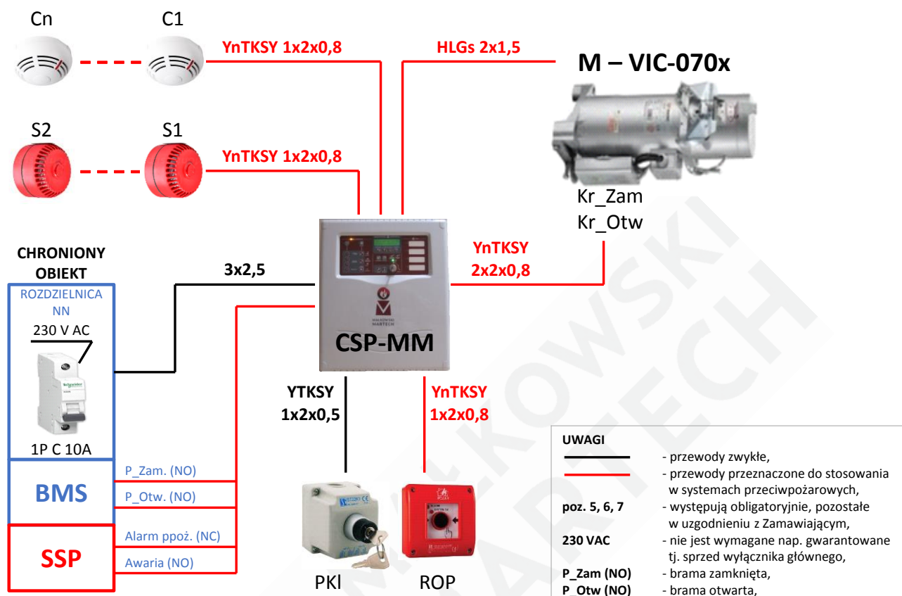
Rys. 13 – Układ sterowania MARC-R z napędem zewnętrznym 24 V DC wariant I – zamykanie / otwieranie napędem, wariant II – zamykanie przeciwwagą, otwieranie napędem
