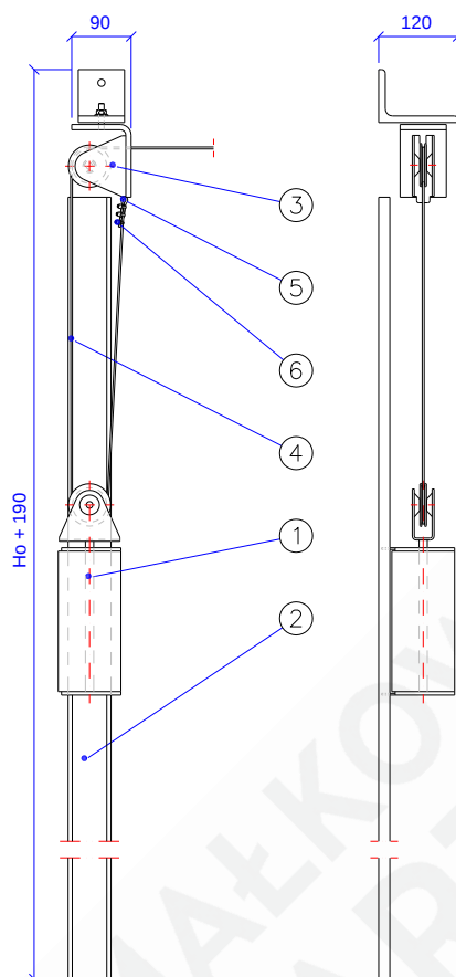
Rys. 6 – MARC-R60-01.05.00 [Zespół przeciwcieżaru]
