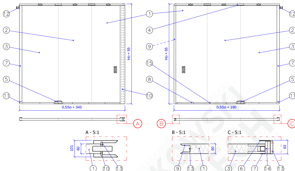
Rys. 2 – MARC-R60-01.01.00 [Skrzydła bramy]
