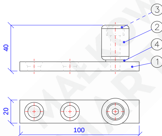
Rys. 7 – MARC-R60-01.06.00 [Prowadnik dolny]
