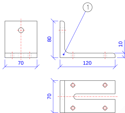
Rys. 4 – MARC-R60-01.03.00 [Wspornik toru jezdnego]
