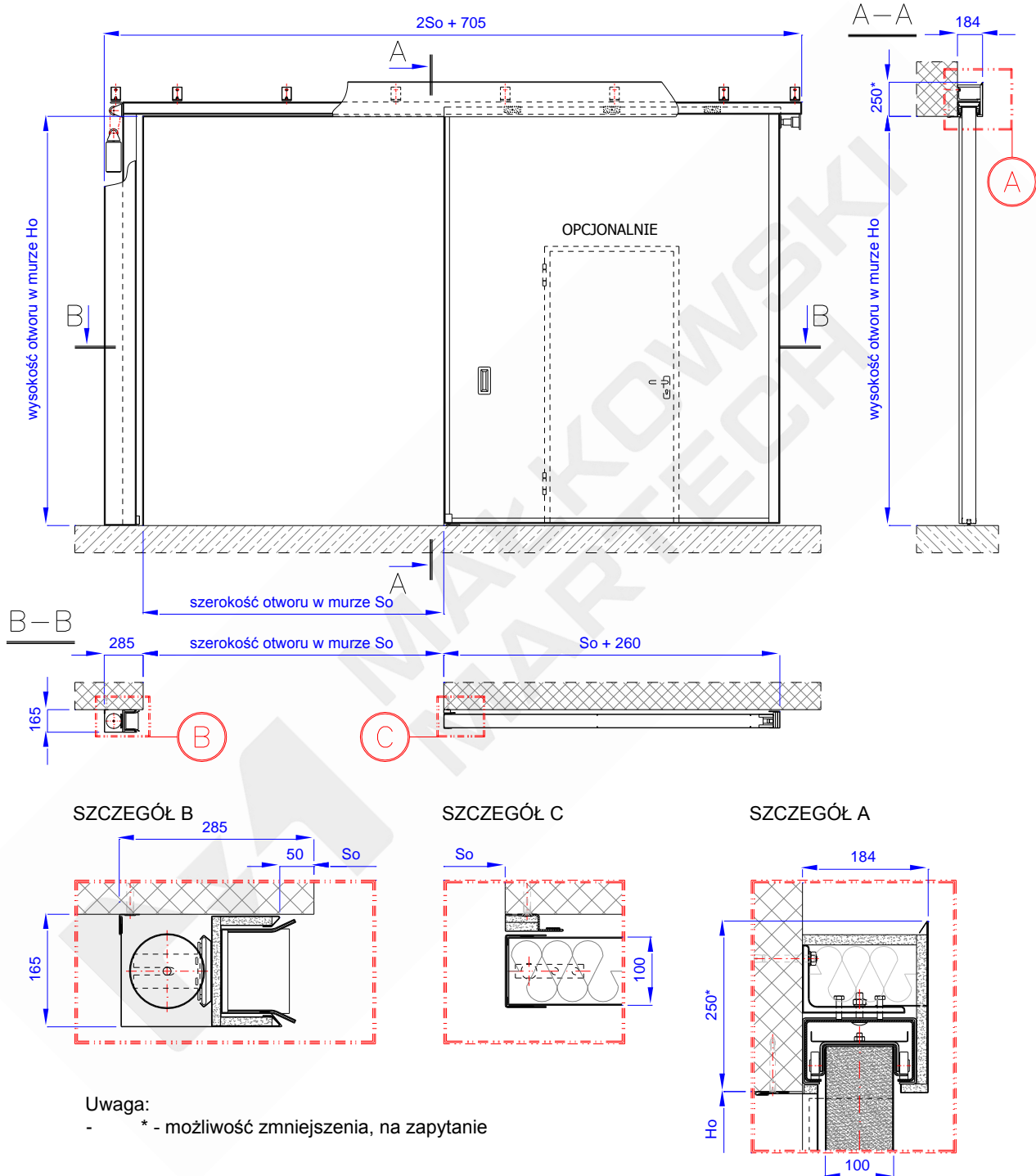
Rys. 1 – Przeciwożarowa brama przesuwna, jednoskrzydłowa typu MARC-P EI120
