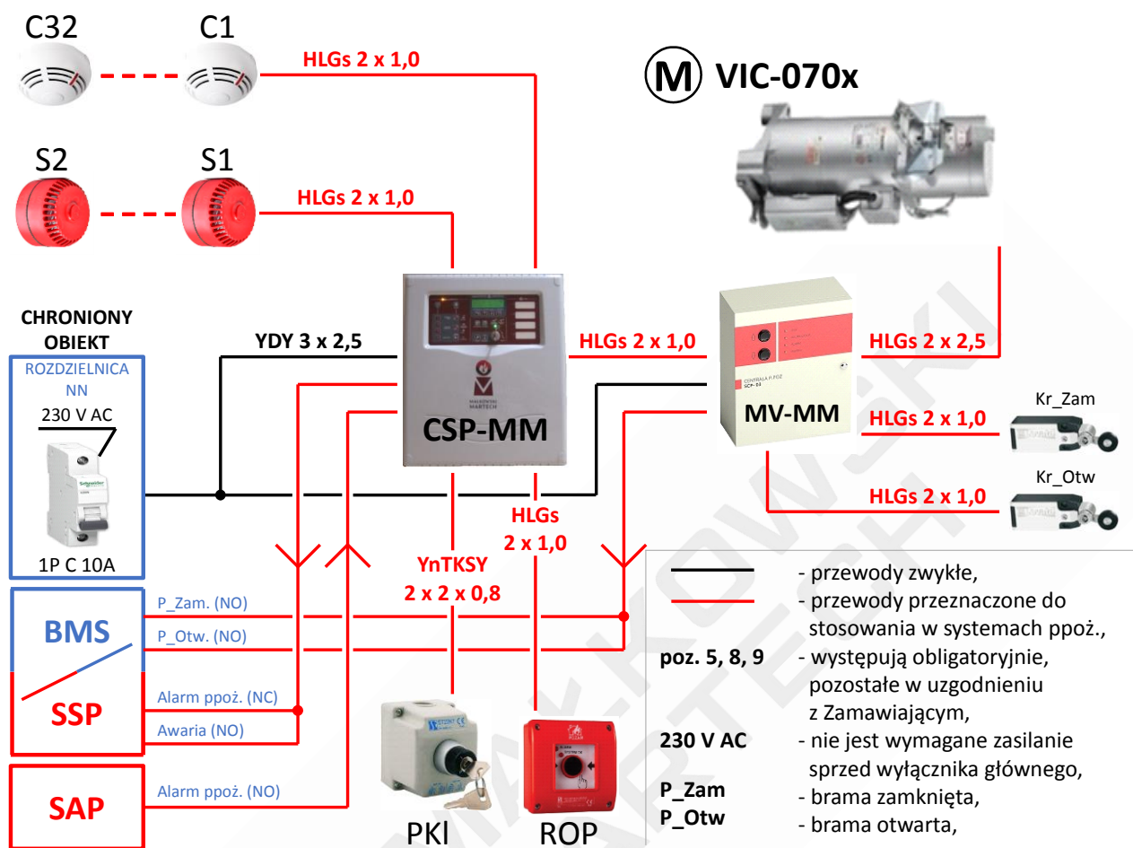
Schemat 2 – Układ sterowania MARC-r z napędem zewnętrznym 24 V DC
