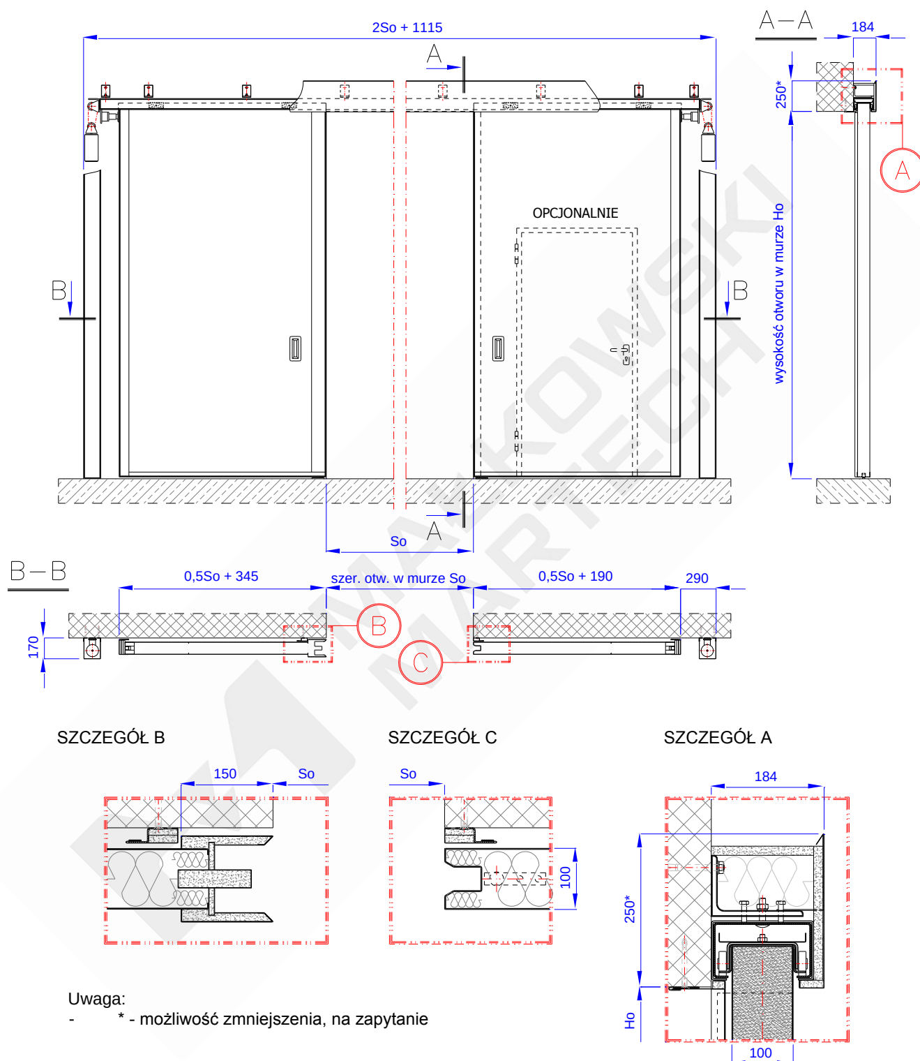
Rys. 1 – Przeciwpowozarowa brama rozsuwana typu MARC-R EI120
