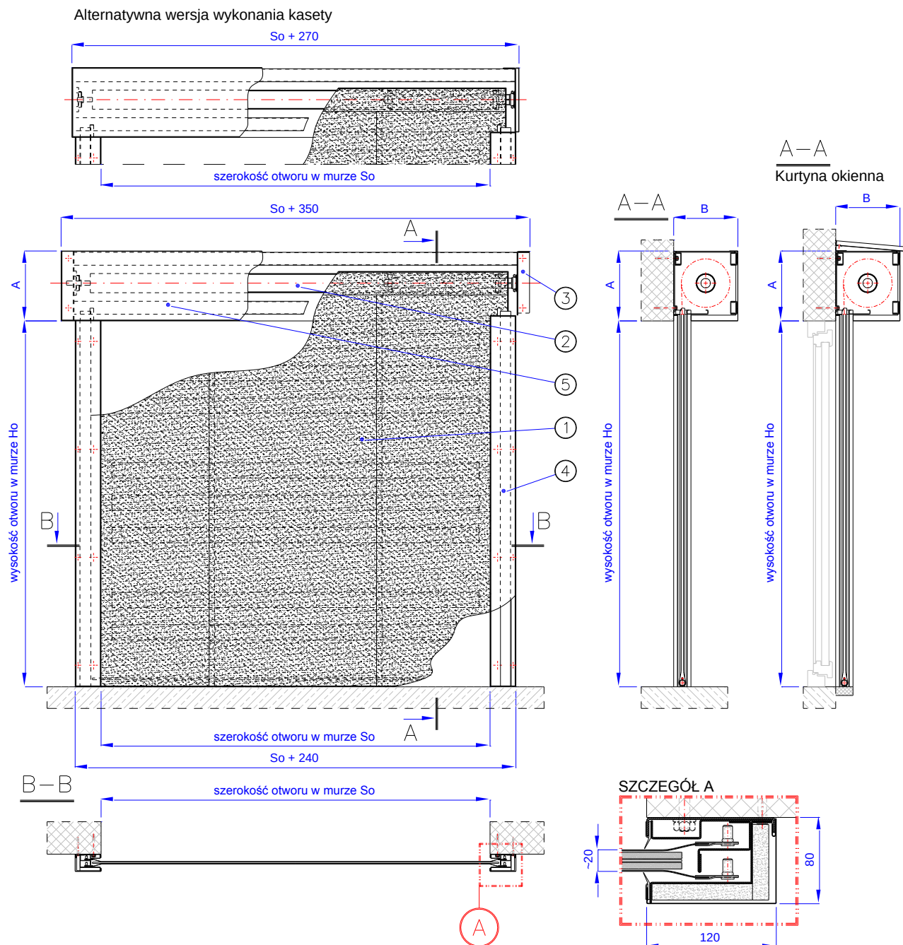
Rys. 2 - Przeciwpożarowa brama kurtynowa typu MARC-Ok EI120
