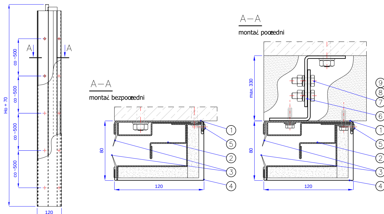
Rys. 9 - MARC-Ok120-01.04.00 [Prowadnica]
