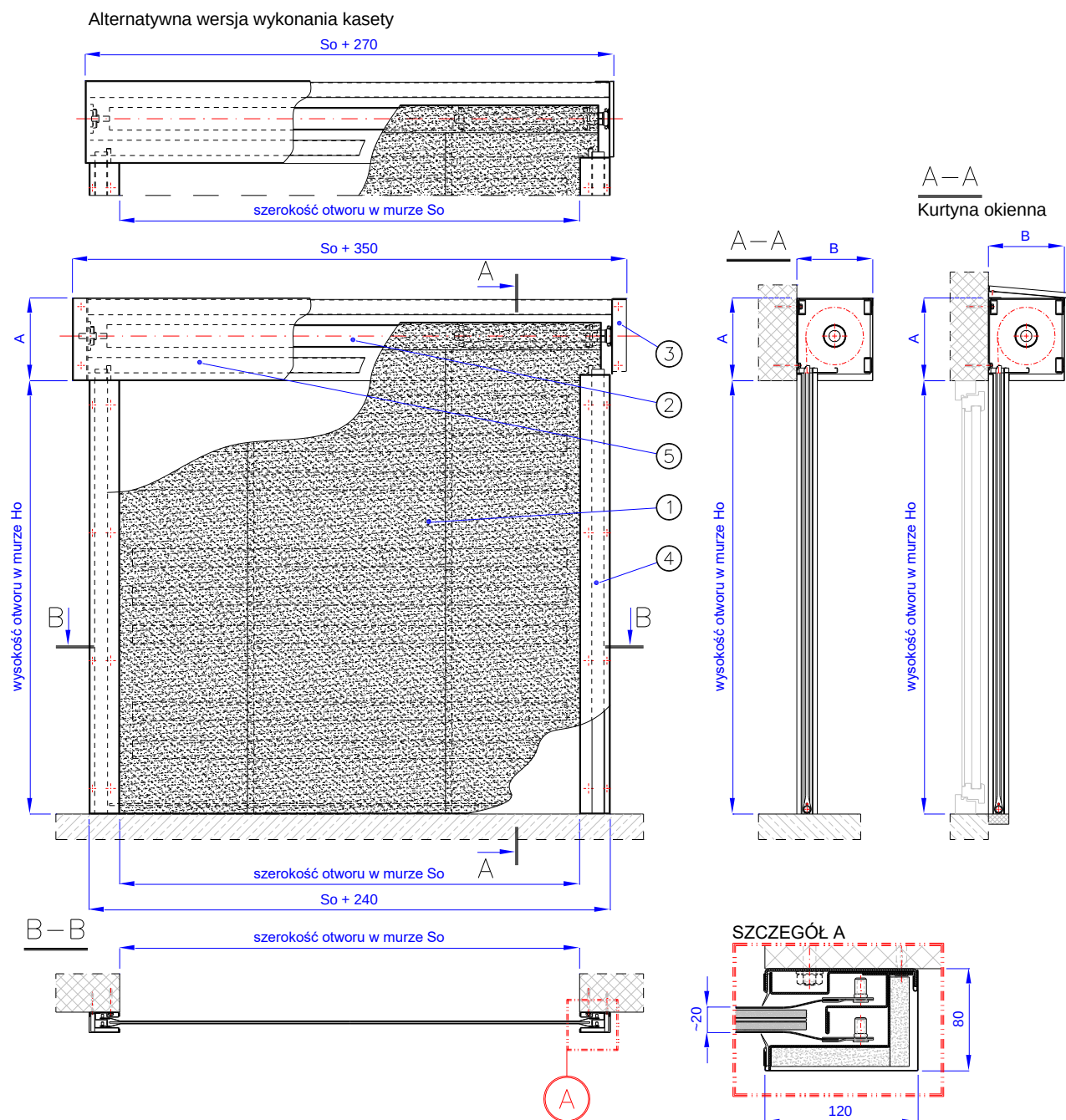
Rys. 2 - Przeciwpowozarowa brama kurtynowa typu MARC-Ok EI120
