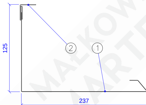
Rys. 12 – MARC-P(1)60-01.10.00 [Osłona modułu przedniego]
