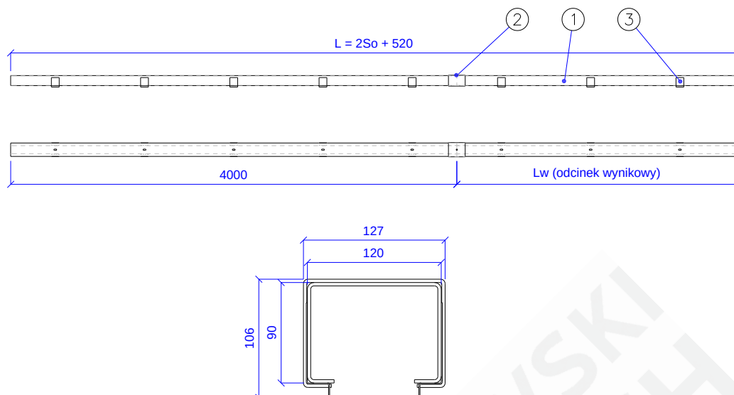
Rys. 4 – MARC-P(1)60-01.02.00 [Tor jezdny]
