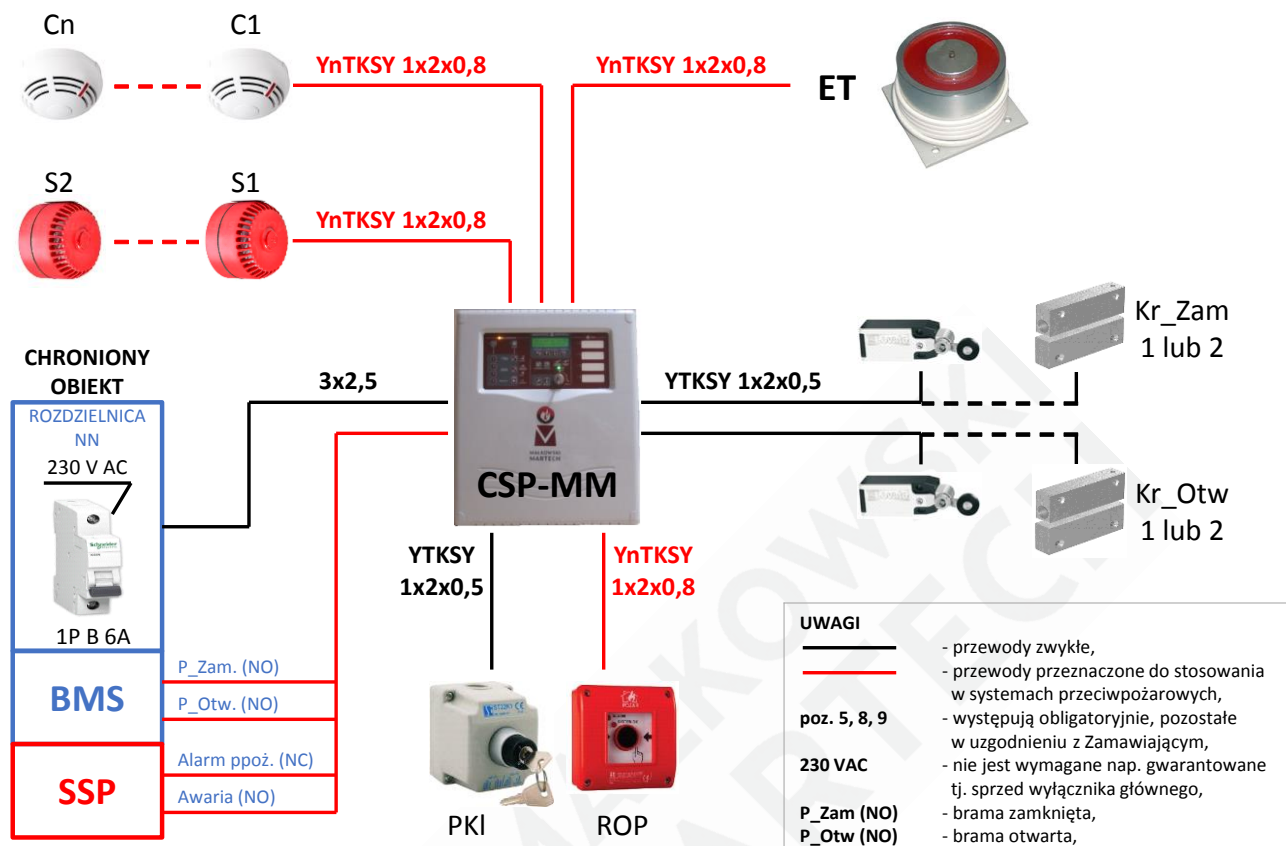
Rys. 13 – Układ sterowania MARC-P1 z trzymaczem elektromagnetycznym
