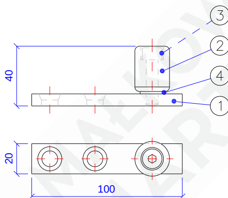
Rys. 8 – MARC-P(1)60-01.06.00 [Prowadnik dolny]
