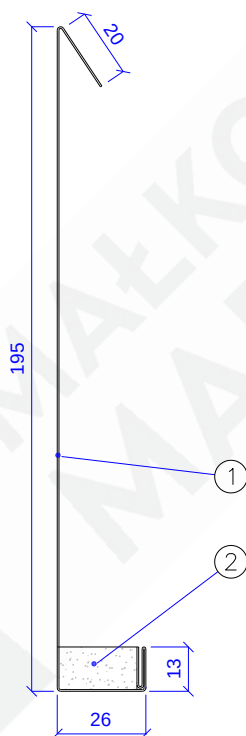
Rys. 11 – MARC-P(1)60-01.09.00 [Osłona toru jezdnego]
