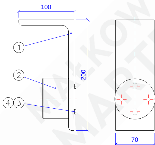
Rys. 9 – MARC-P(1)60-01.07.00 [Zespół trzymacza elektromagnetycznego]
