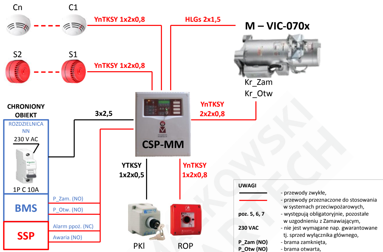
Rys. 14 – Układ sterowania MARC-P1 z napędem zewnętrznym 24 V DC
