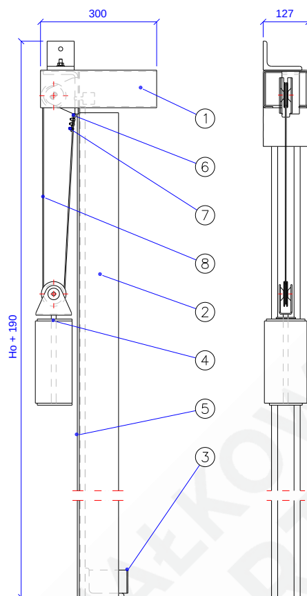
Rys. 7 – MARC-P(1)60-01.05.00 [Moduł przedni]
