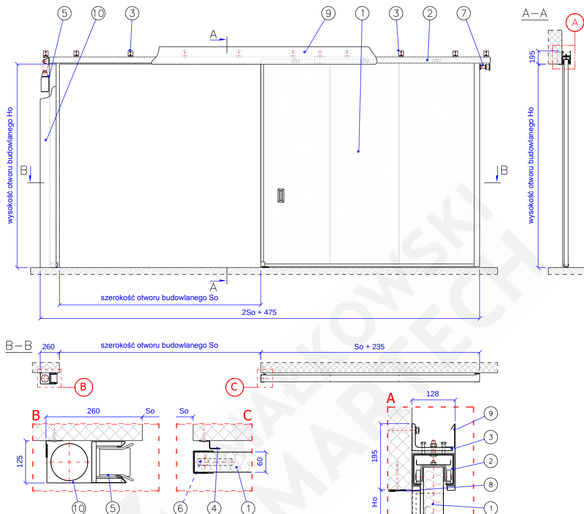
Rys. 1 – MARC-P(1)60-01.00.00 [Przeciwpożarowa brama przesuwna jednoskrzydłowa typu MARC-P1 EI60]
