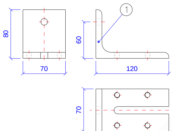
Rys. 5 – MARC-P(1)60-01.03.00 [Wspornik toru jezdnego]
