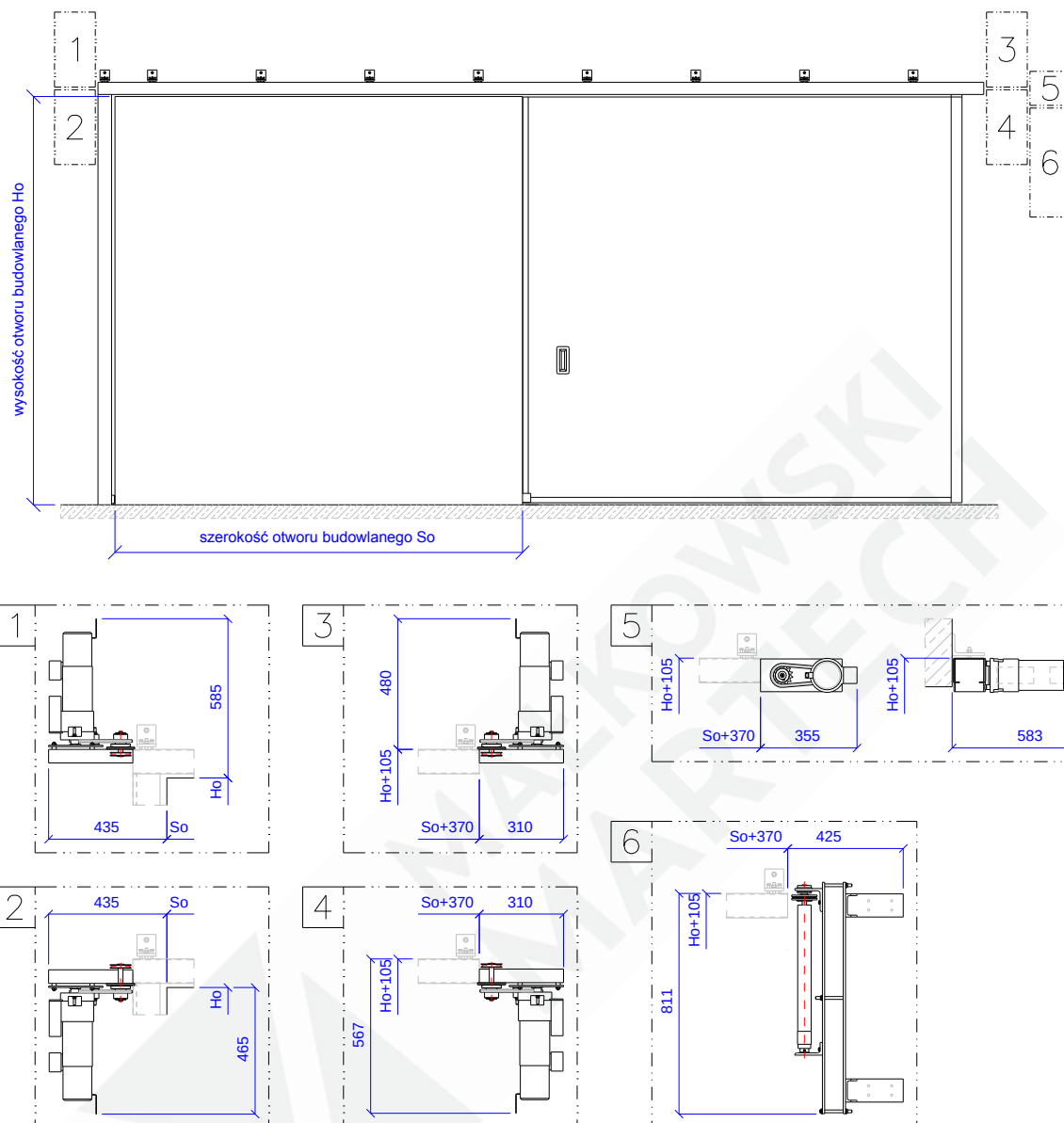
Rys. 3 – Warianty montażu napędu elektrycznego typu VIC
