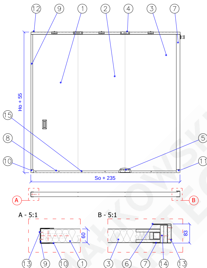
Rys. 2 – MARC-P(1)60-01.01.00 [Skrzydło bramy]
