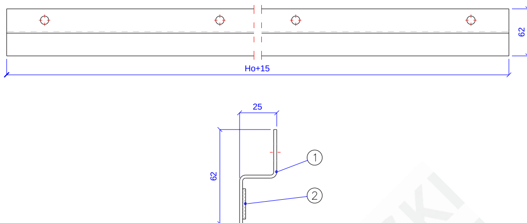
Rys. 6 – MARC-P(1)60-01.04.00 [Przymyk naścienny]
