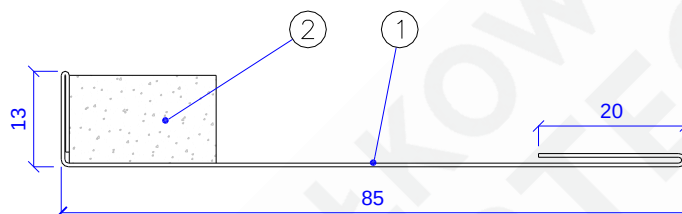
Rys. 10 – MARC-P(1)60-01.08.00 [Osłona nadproża]
