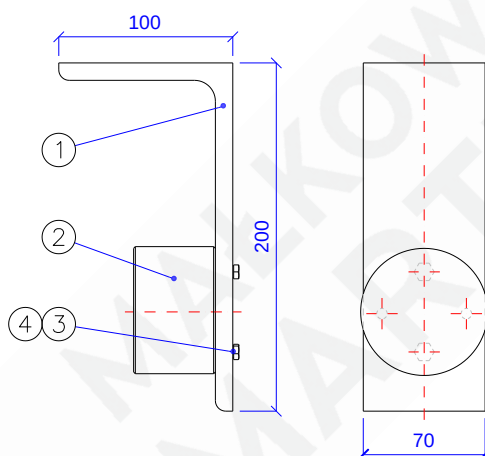
Rys. 9 – MARC-P(1)120-01.07.00 [Zespół trzymacza elektromagnetycznego]
