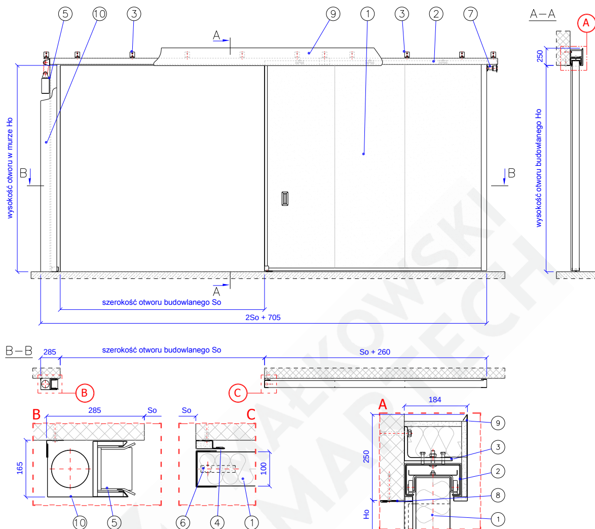
Rys. 1 – MARC-P120-01.00.00 [Przeciwpożarowa brama przesuwna jednoskrzydłowa typu MARC-P1 EI120]
