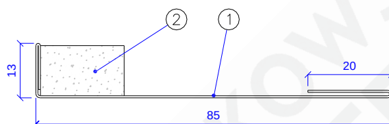
Rys. 10 – MARC-P(1)120-01.08.00 [Osłona nadproża]
