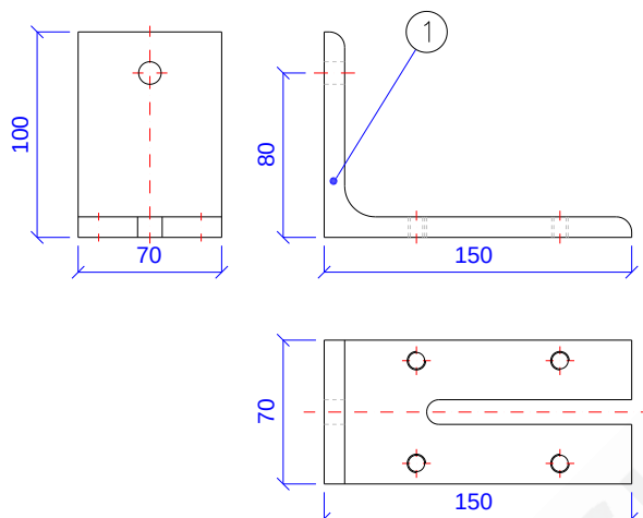
Rys. 5 – MARC-P(1)120-01.03.00 [Wspornik toru jezdnego]
