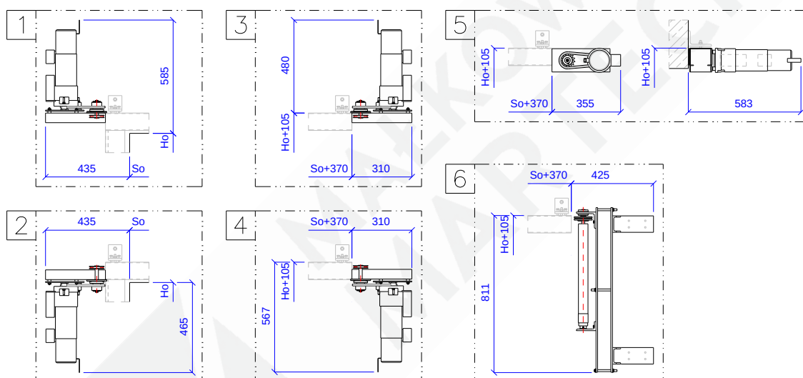
Rys. 3 – Warianty montażu napędu elektrycznego typu VIC
