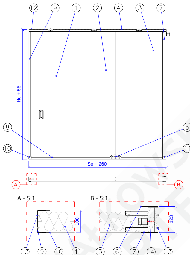
Rys. 2 – MARC-P(1)120-01.01.00 [Skrzydło bramy]
