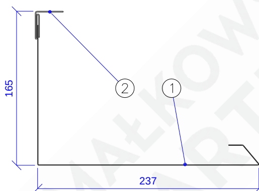
Rys. 12 – MARC-P(1)120-01.10.00 [Osłona modułu przedniego]
