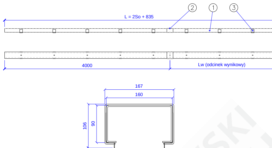
Rys. 4 – MARC-P(1)120-01.02.00 [Tor jezdny]
