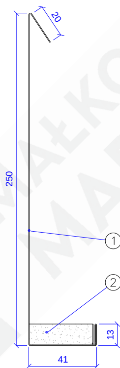
Rys. 11 – MARC-P(1)120-01.09.00 [Osłona toru jezdnego]
