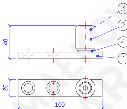
Rys. 8 – MARC-P(1)120-01.06.00 [Prowadnik dolny]
