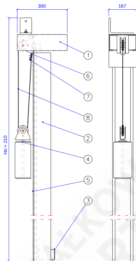
Rys. 7 – MARC-P(1)120-01.05.00 [Moduł przedni]
