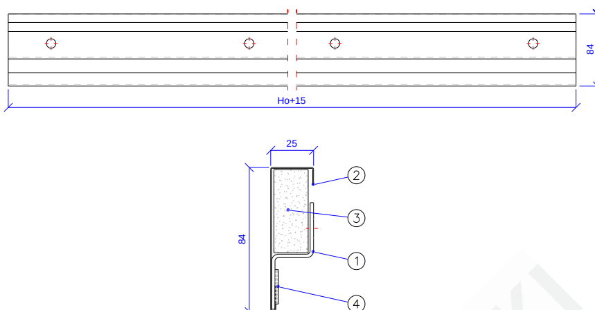
Rys. 6 – MARC-P(1)120-01.04.00 [Przymyk naścienny]
