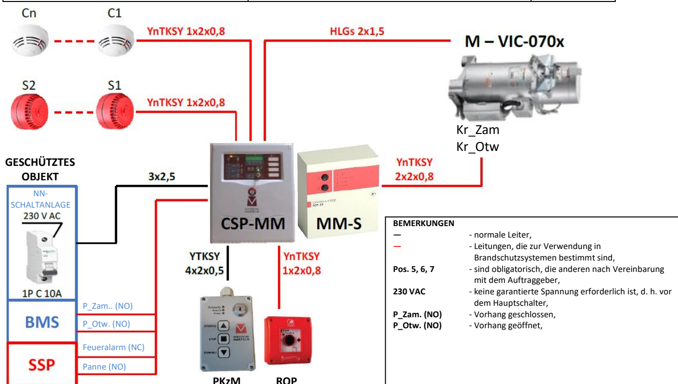
Abb. 9 – MARC-Ok Steuerung mit externem 24 V DC Antrie
