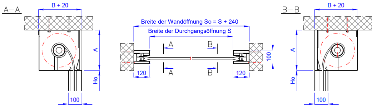
Abb. 2 – Schutztür Typ MARC-Ok EI60 Einbau im Flur (Nische) - fehlender Türsturz und beide Traufen
