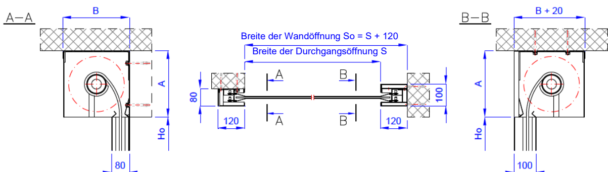
Abb. 3 – Brandschutzvorhang Typ MARC-Ok EI60 gemischter Einbau - fehlender Türsturz und Traufen auf der rechten Seite
