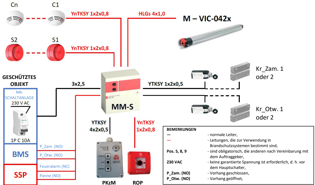
Abb. 8 – MARC-Ok-Steuerung mit internem (Rohr-)Antrieb 230 V AC mit Wechselrichter
