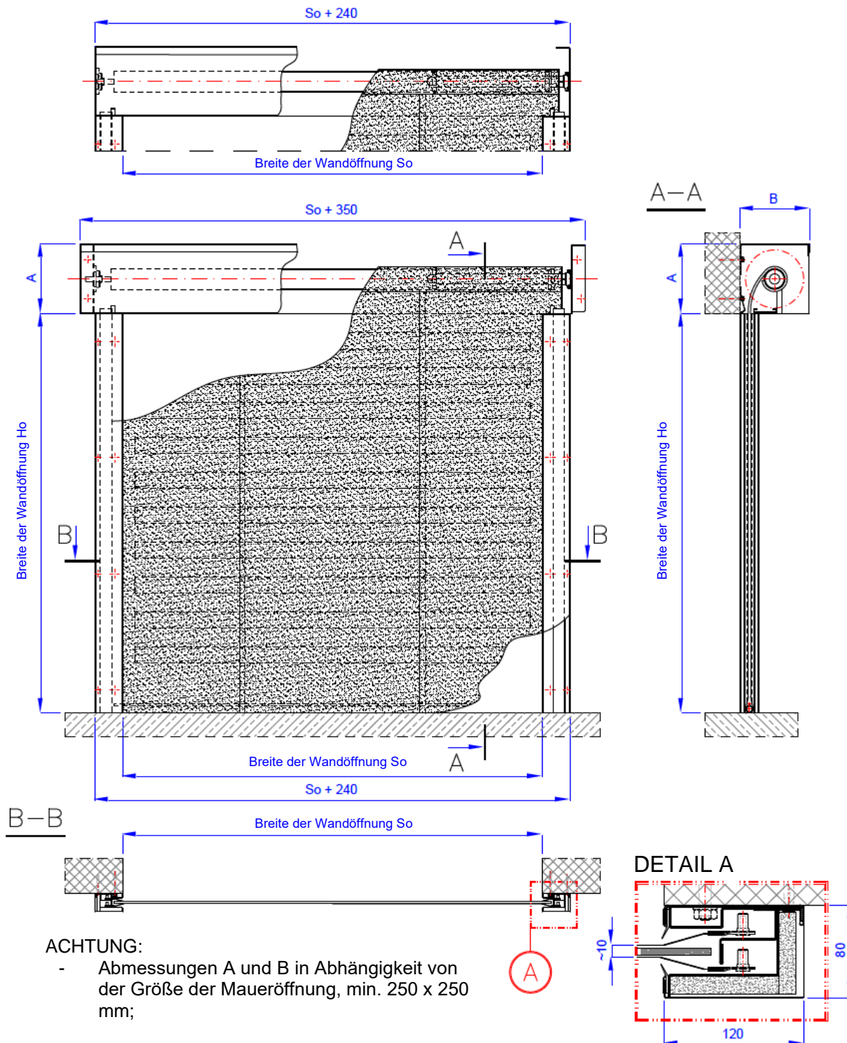
Abb. 1 – Brandschutzvorhang Typ MARC-Ok EI60 mit elektrischem Innenantrieb
