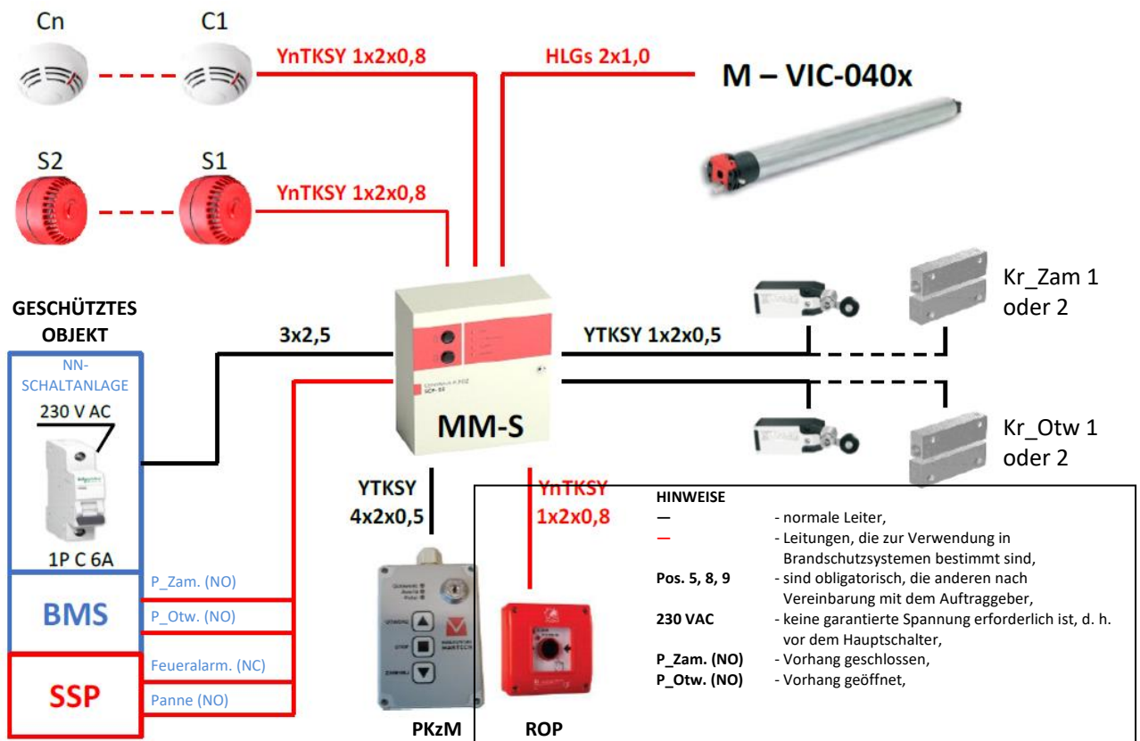
Abb. 5 – MARC-Ok-Steuerungssystem mit internem (rohrförmigem) Antrieb 24 V DC
