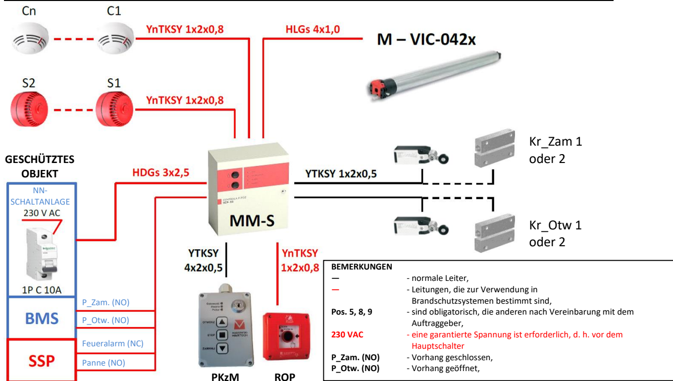
Abb. 7 – MARC-Ok-Steuerung mit internem (röhrenförmigem) Antrieb 230 V AC garantierte Spannung
