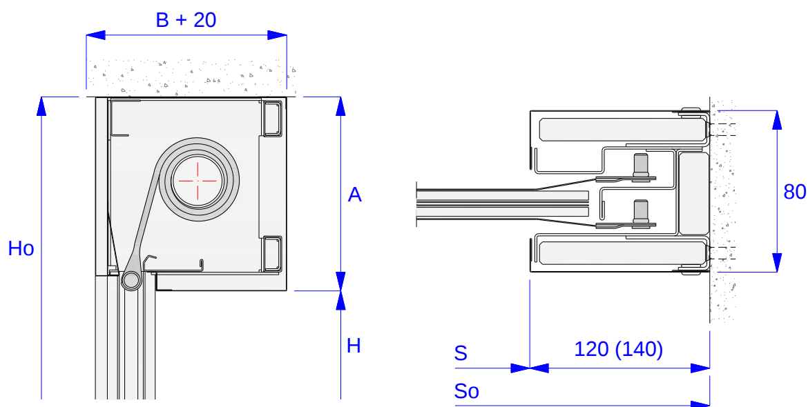
Rys. 4 – ISOiK-Ok60-01.04 Przeciwpółarowa brama kurtynowa typu MARC-Ok + EI60 – montaż korytarzowy (wnętkowy)
