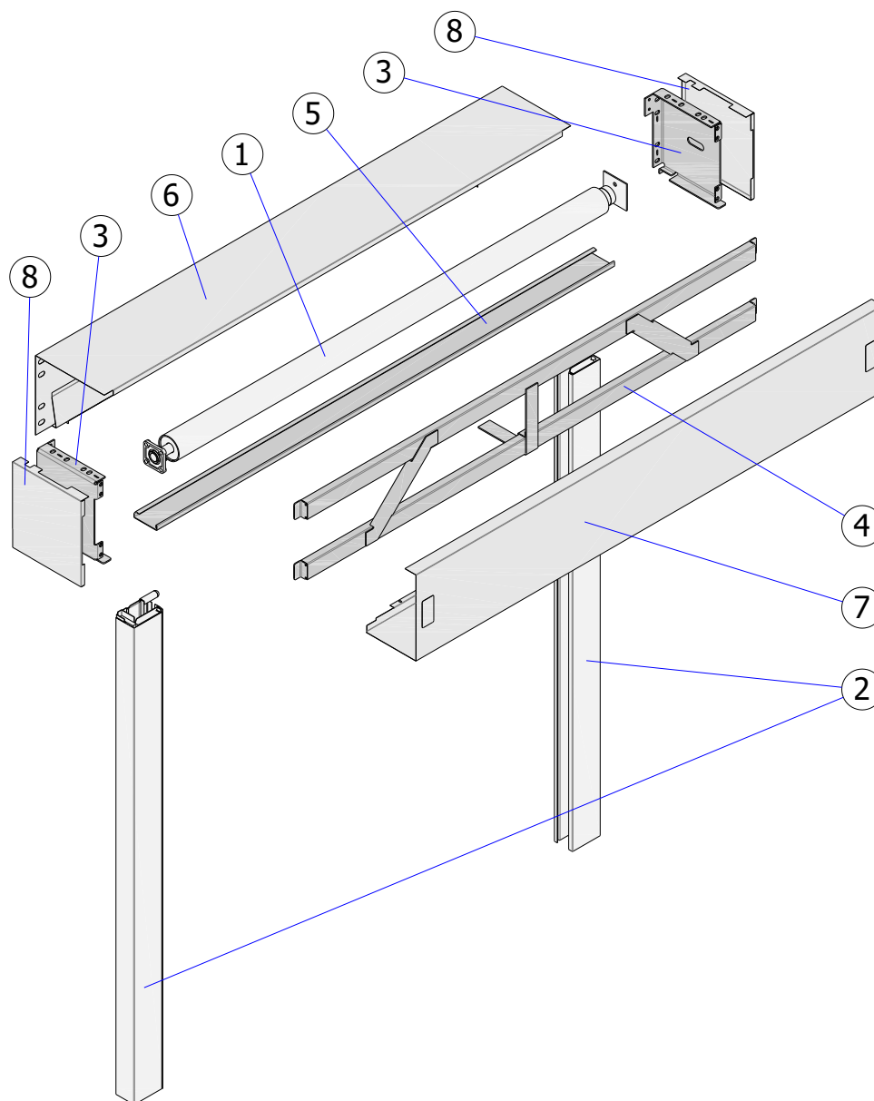
Rys. 2 - ISOiK-Ok60-01.02 Przeciwpożarowa brama kurtynowa MARC-Ok + EI60 z napędem wewnętrznym
