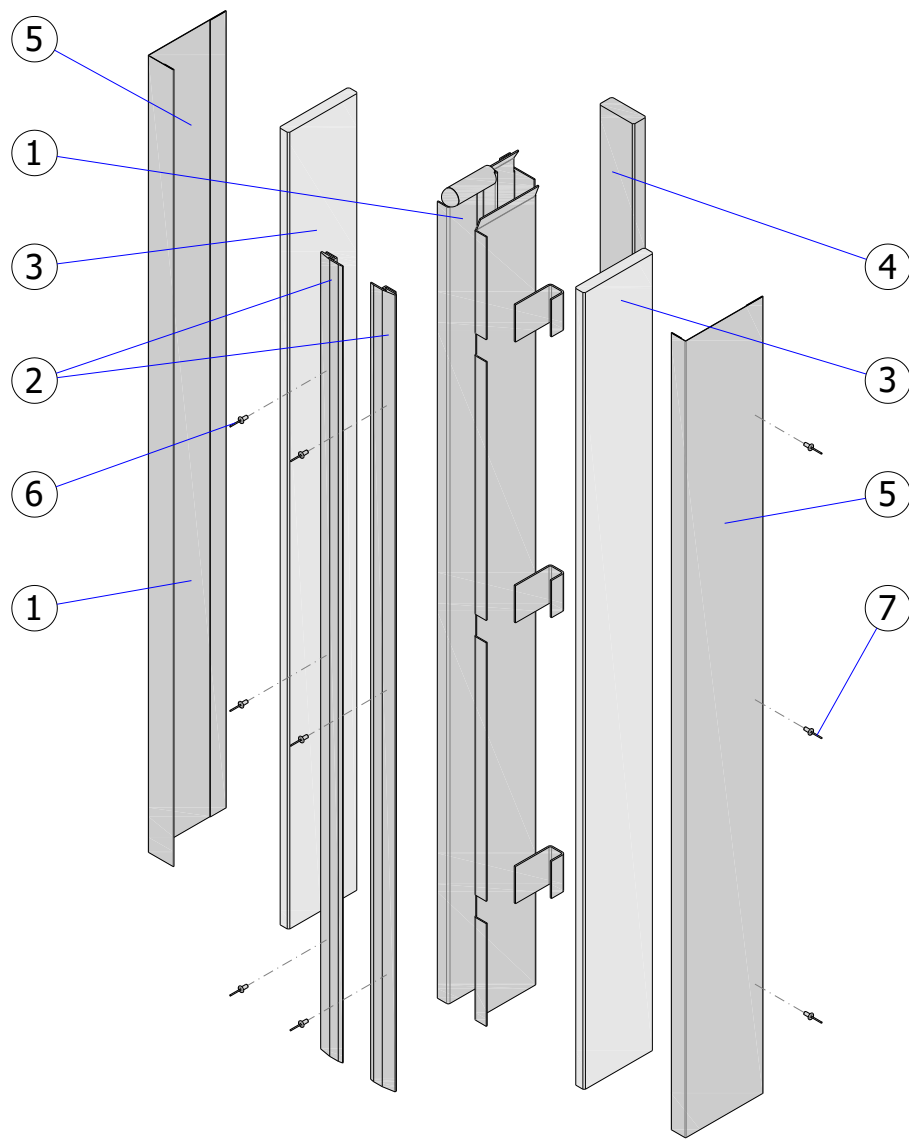
Rys. 22 – ISOiK-Ok60-01.22 [Prowadnica – wersja korytarzowa]
