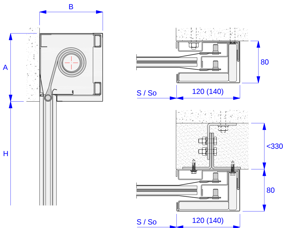
Rys. 3 - ISOiK-Ok60-01.03 Przeciwpółarowa brama kurtynowa typu MARC-Ok + EI60 – montaż naścienny
