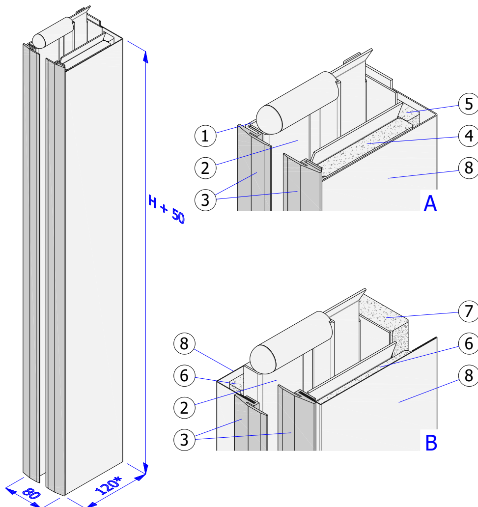
Rys. 7 - ISOiK-Ok60-01.07 [Prowadnica, A – wersja ppoż., naścienna, B – wersja ppoż., korytarzowa]
