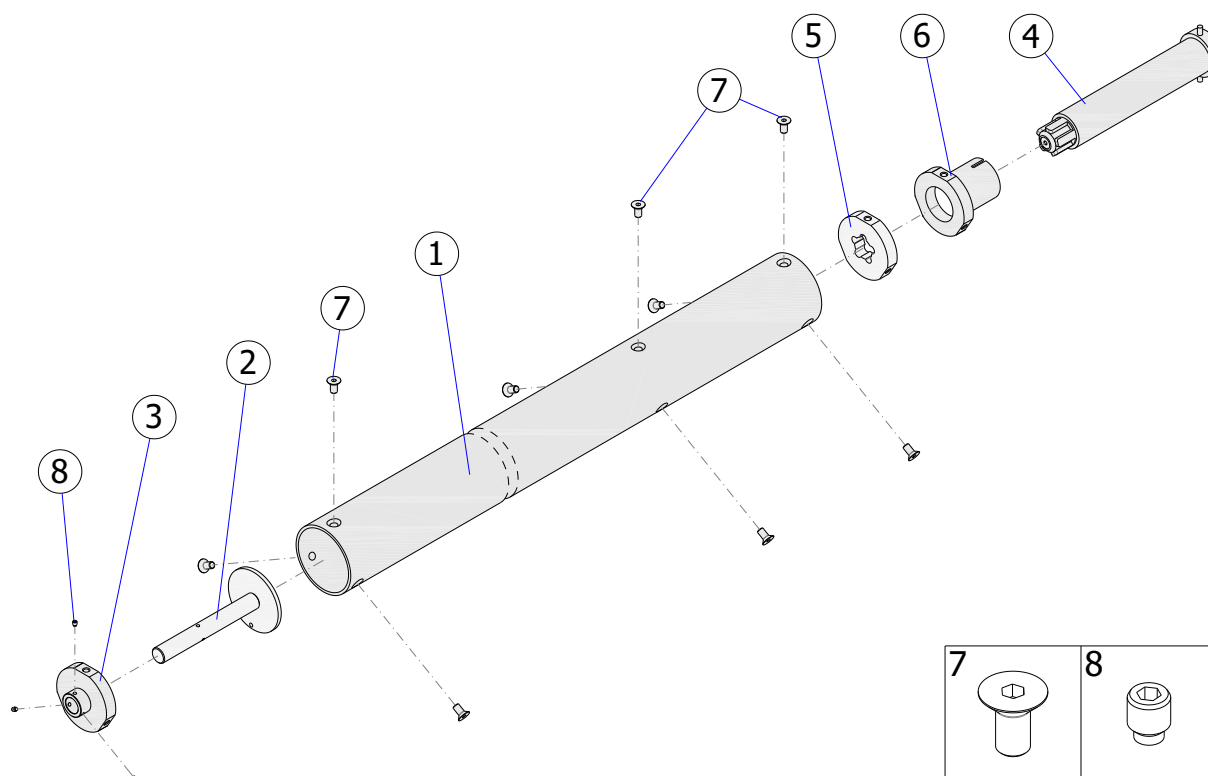
Rys. 19 – ISOiK-Ok30-01.19 [Wał nawojowy z napędem wewnętrznym]
