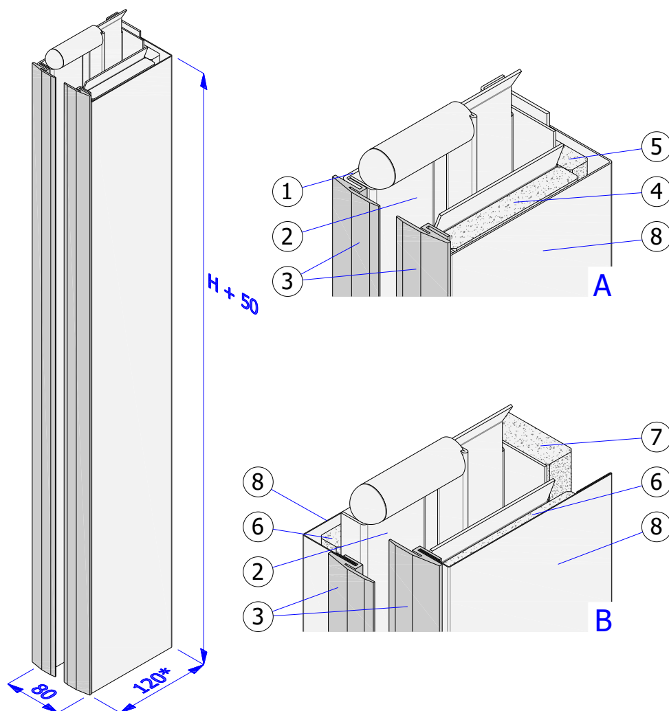
Rys. 7 - ISOiK-Ok30-01.07 [Prowadnica, A – wersja ppoż., naścienna, B – wersja ppoż., korytarzowa]
