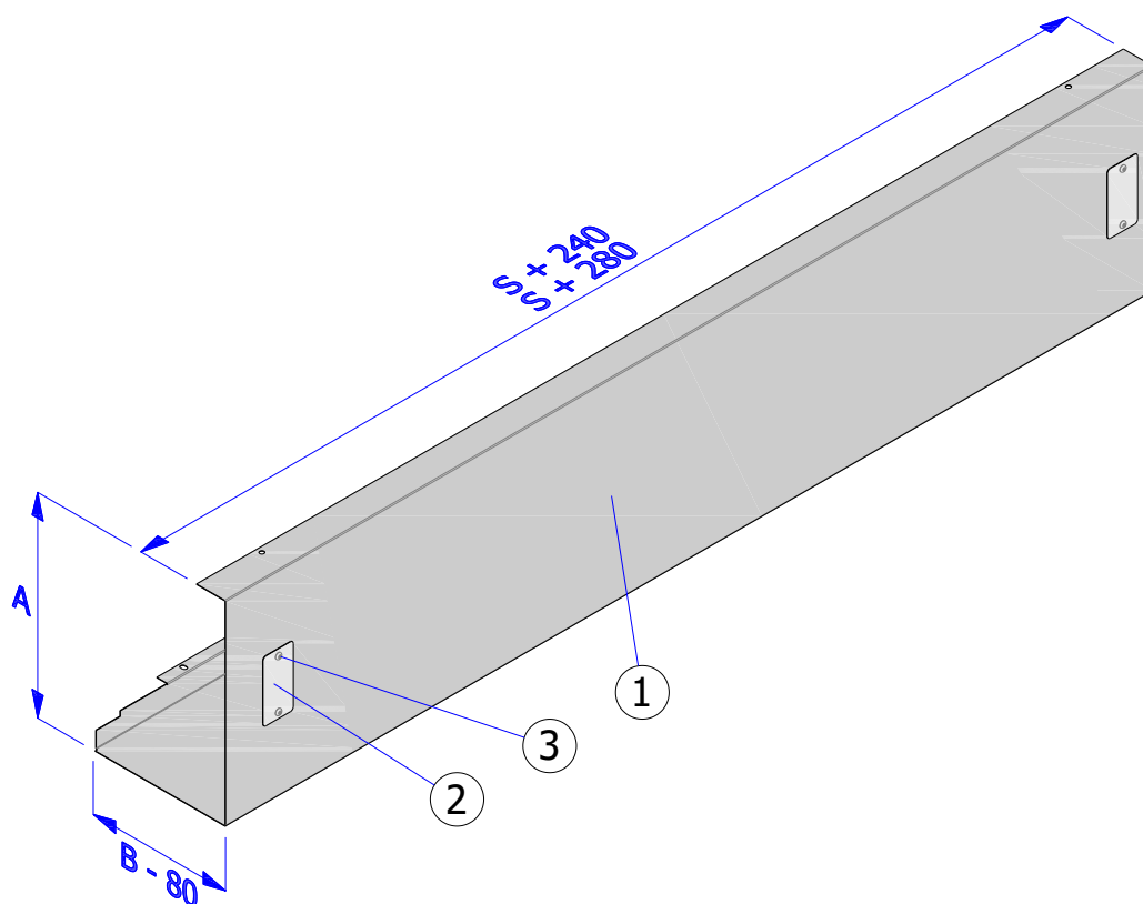
Rys. 13 - ISOiK-Ok30-01.13 [Osłona czołowa] 1 – Profil osłony, 2 – Zaślepka otworu rewizyjnego
