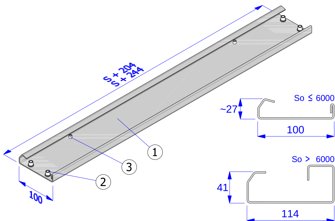
Rys. 11 - ISOiK-Ok30-01.11 [Listwa dopychająca] 1 – Profil listwy, 2 – Nitonakrętka M6, 3 – Nitonakrętka M5
