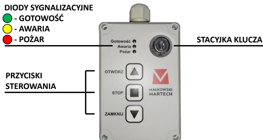
Rys. 1 - Panel wyniesiony sterowania przeciwpożarowej bramy kurtynowej typu MARC-Ok
