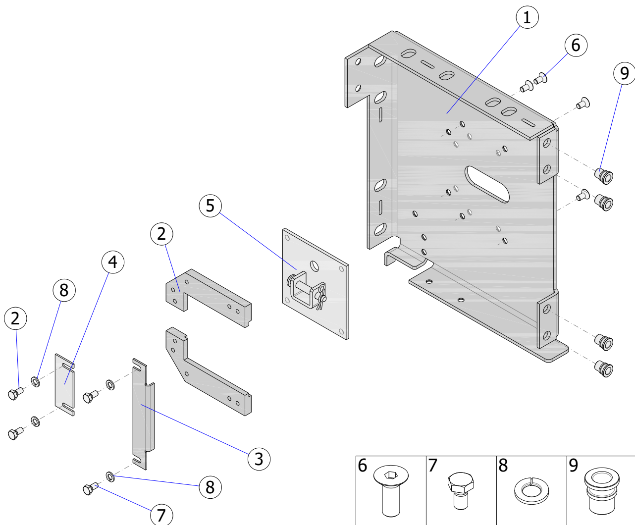
Rys. 23 – ISOiK-Ok30-01.23 [Wspornik wału – strona napędowa]
