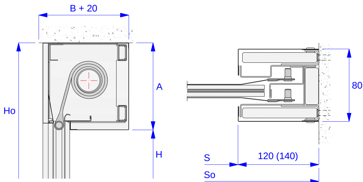
Rys. 4 –ISOiK-Ok30-01.04 Przeciwpółarowa brama kurtynowa typu MARC-Ok + EI30 – montaż korytarzowy (wnętkowy)
