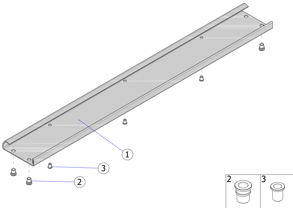
Rys. 26 – ISOiK-Ok30-01.26 [Listwa dopychająca]
