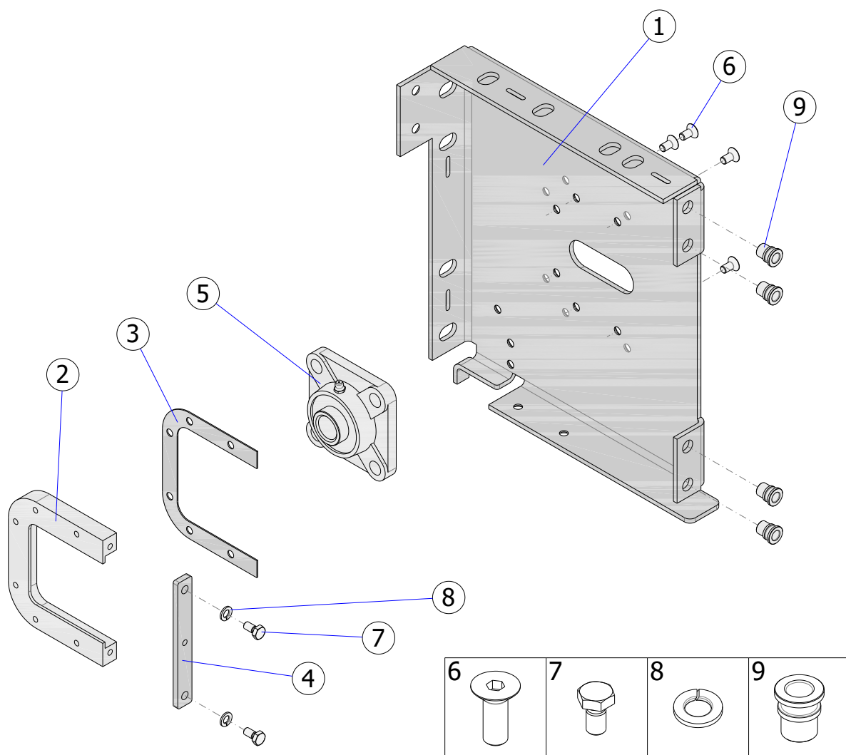
Rys. 24 – ISOiK-Ok30-01.24 [Wspornik wału – strona bierna]
