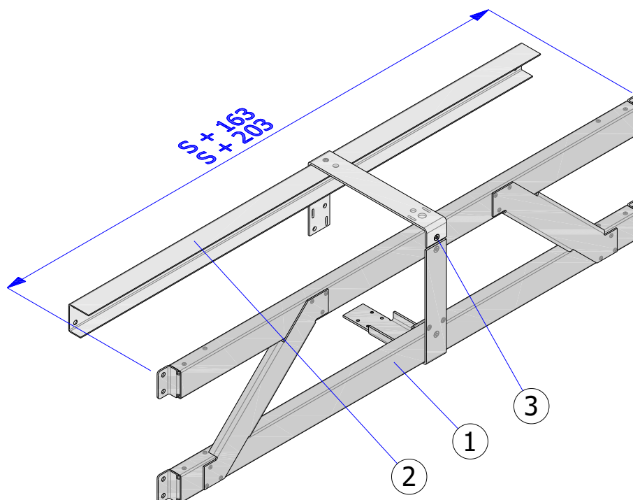
Rys. 10 - ISOiK-Ok30-01.10 [Konstrukcja kratowa z ceownikiem naściennym]
