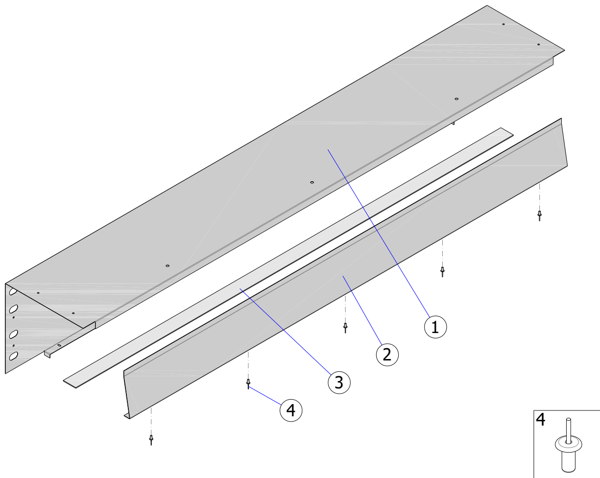
Rys. 27 – ISOiK-Ok30-01.27 [Osłona tylna]
