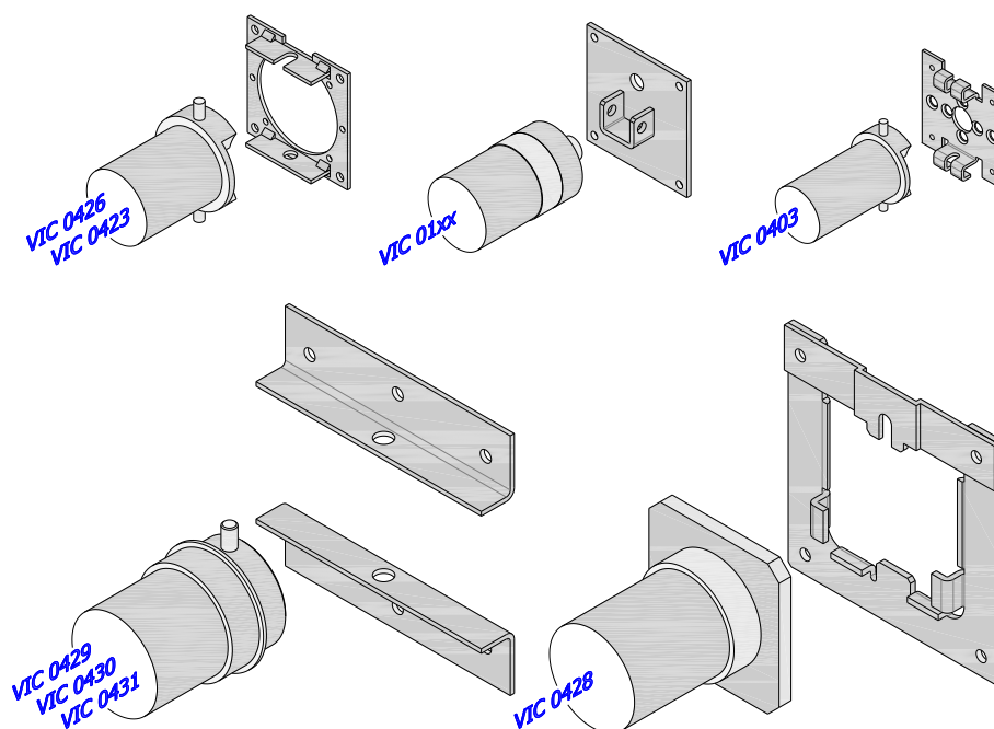
Rys. 9 - ISOiK-Ok30-01.09 [Uchwyty poszczególnych napędów wewnętrznych]
