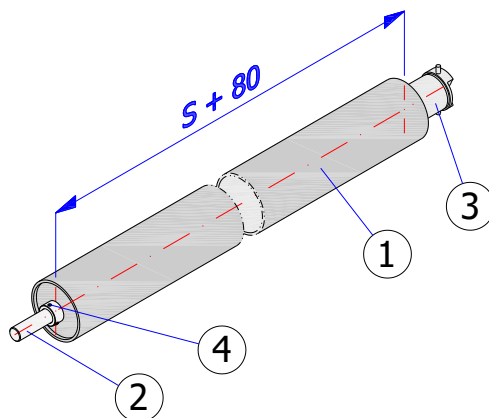
Rys. 5 – ISOiK-Ok30-01.05 [Wał nawojowy z napędem wewnętrznym]
