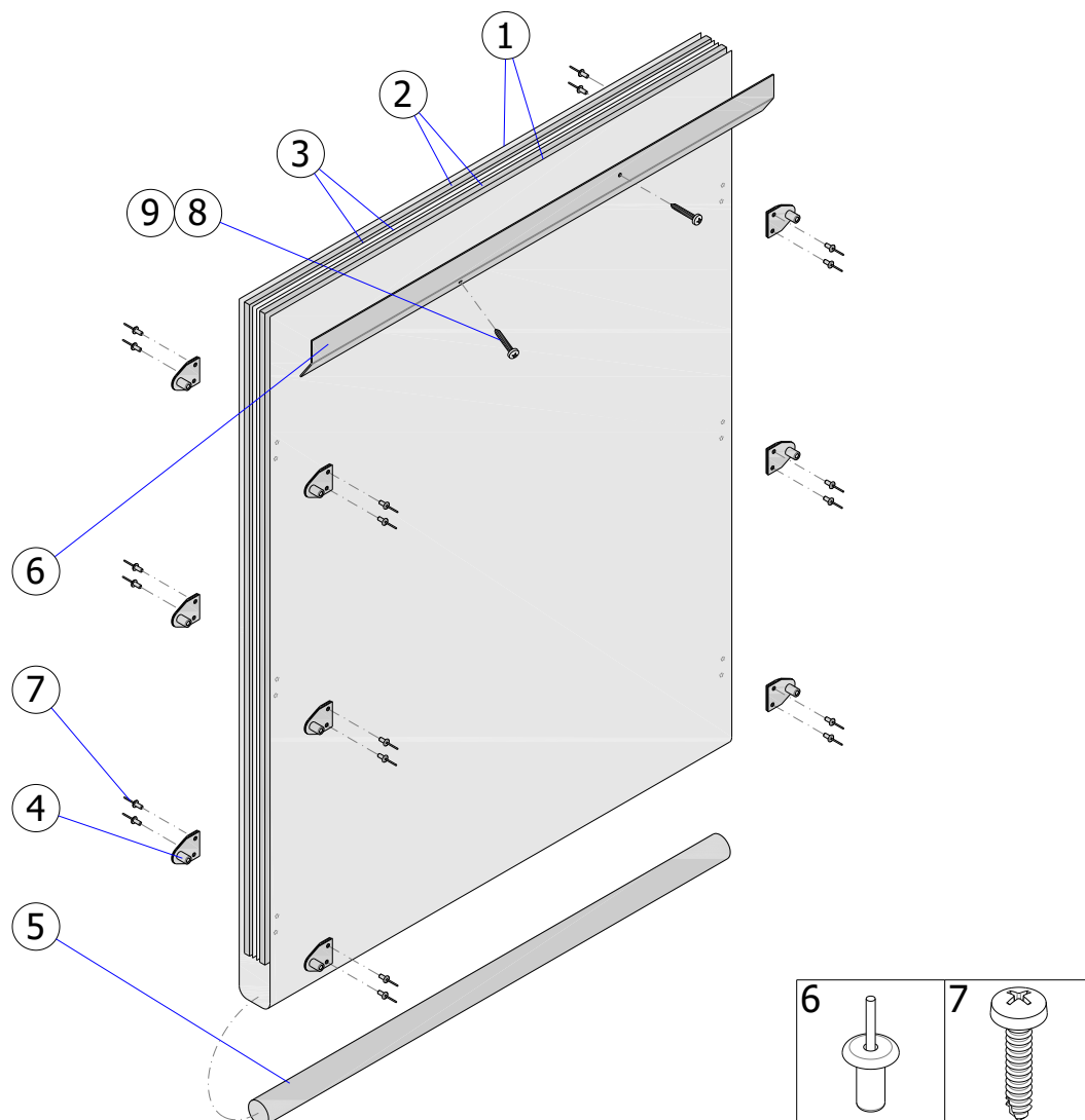
Rys. 20 – ISOiK-Ok30-01.20 [Płaszcz bramy]
