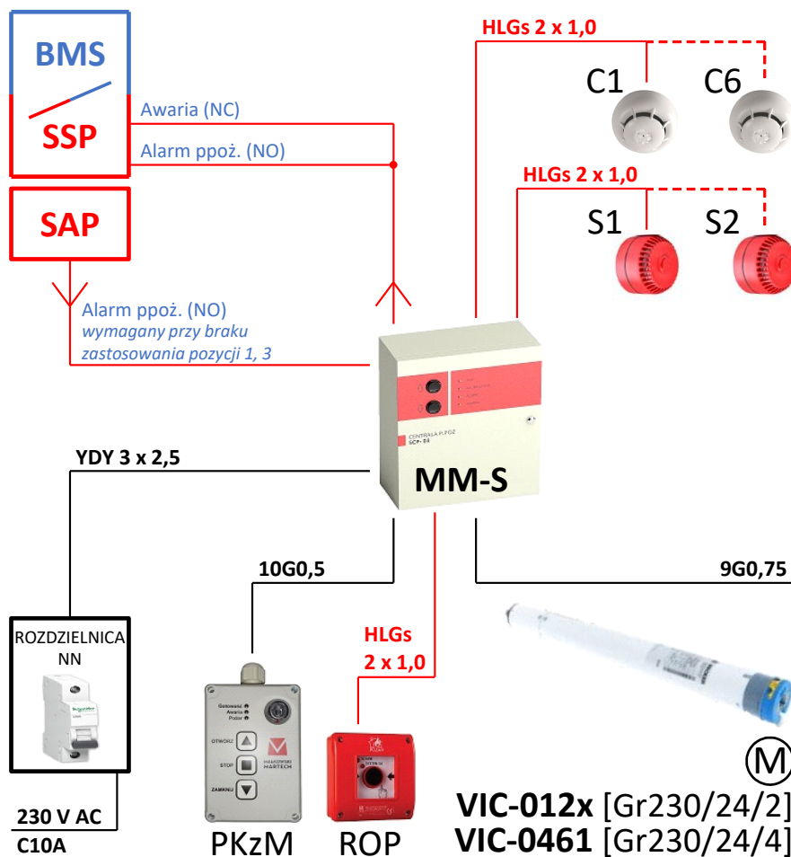
Rys. 16 – Układ sterowania MARC-Ok z napędem wewnętrznym (rurowym) 230 V AC
