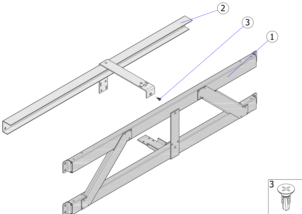
Rys. 25 – ISOiK-Ok30-01.25 [Konstrukcja kratowa z ceownikiem naściennym]
