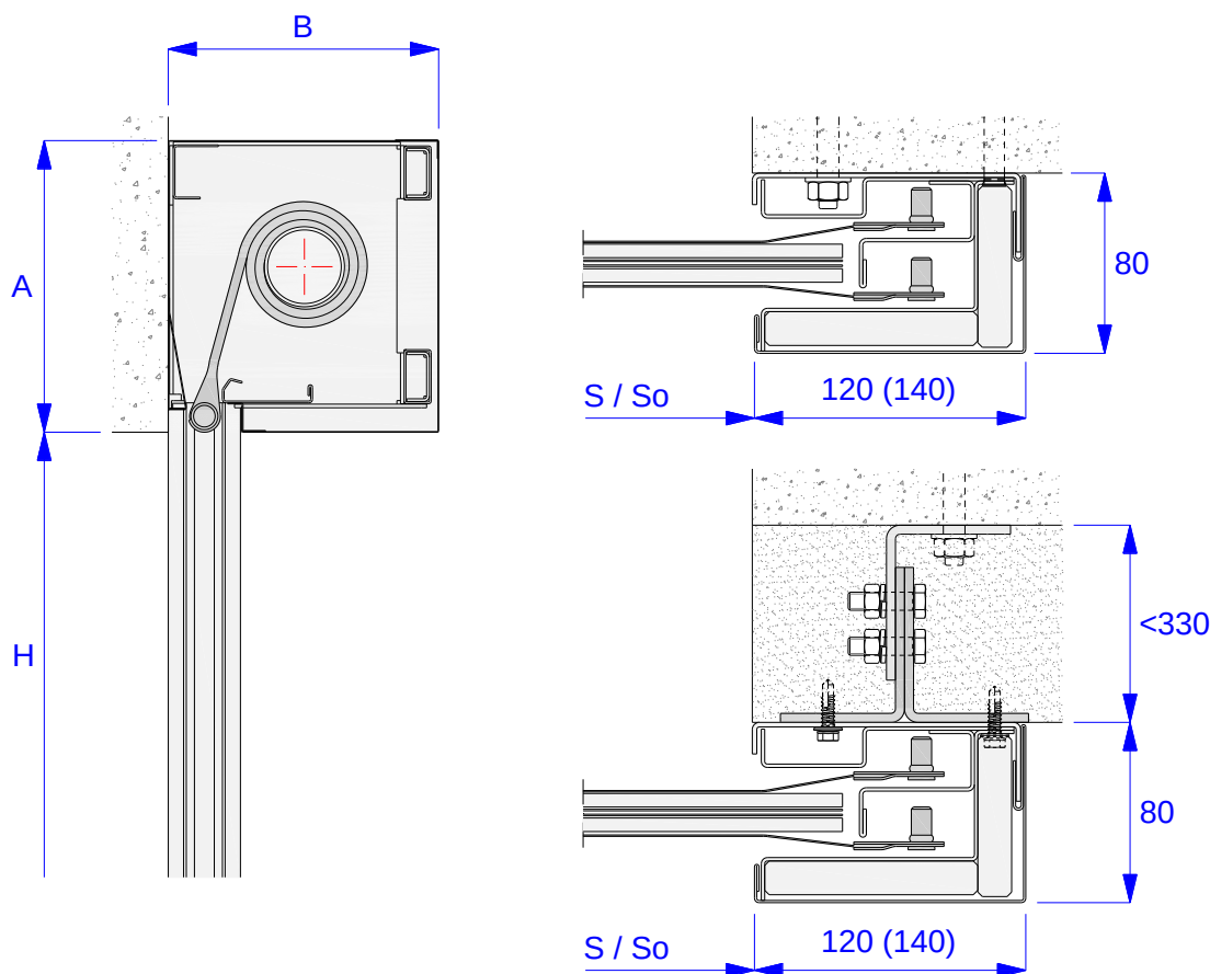
Rys. 3 - ISOiK-Ok30-01.03 Przeciwpółarowa brama kurtynowa typu MARC-Ok + EI30 – montaż naścienny
