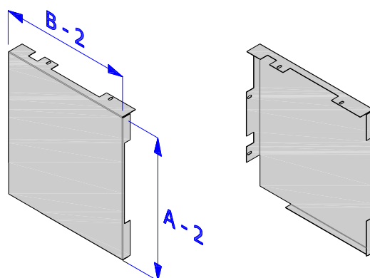
Rys. 14 - ISOiK-Ok30-01.14 [Osłona boczna]
