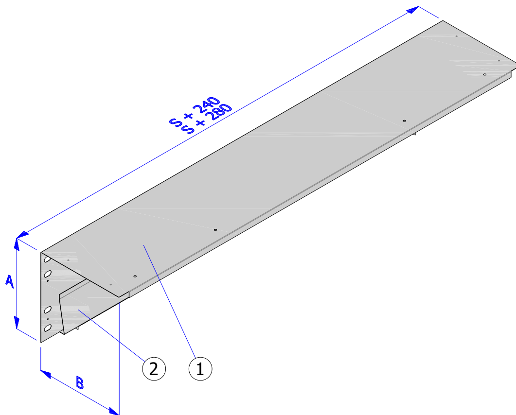
Rys. 12 - ISOiK-Ok30-01.12 [Osłona tylna]
