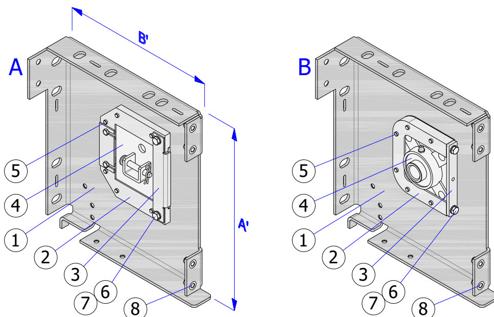
Rys. 8 - ISOiK-Ok30-01.08 [Wspornik wału, A - strona napędowa, B - strona bierna]
