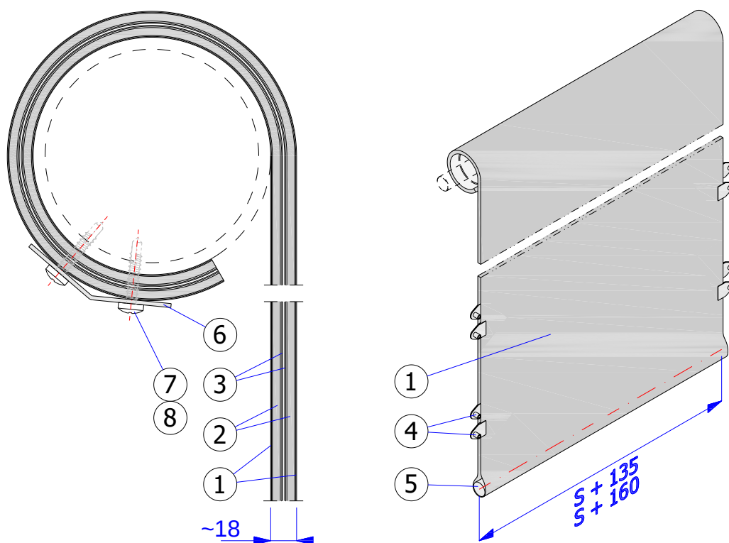
Rys. 6 - ISOiK-Ok30-01.06 [Płaszcz bramy]
