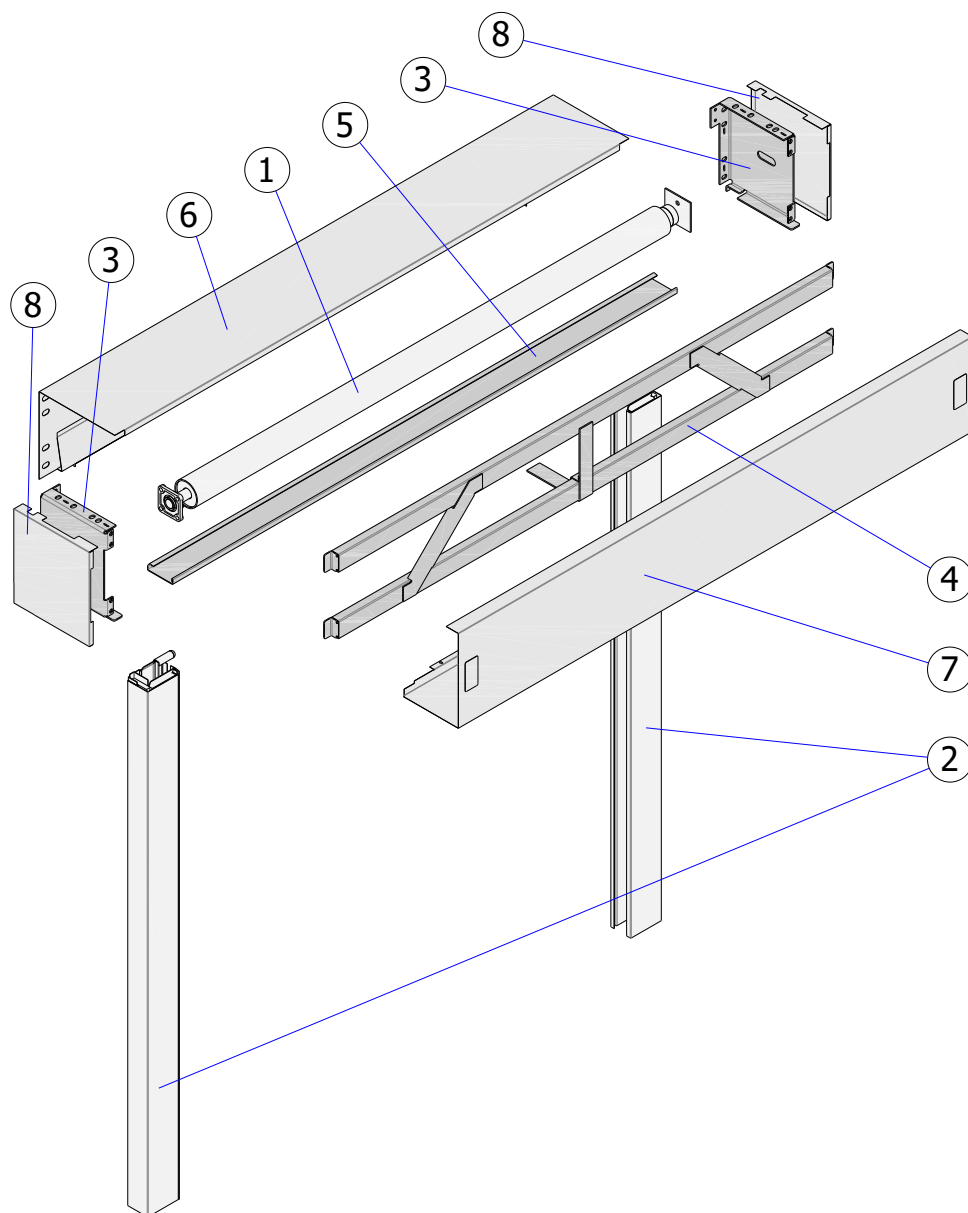
Rys. 2 - ISOiK-Ok30-01.02 Przeciwp0żarowa brama kurtynowa MARC-Ok + EI30 z napędem wewnętrznym
