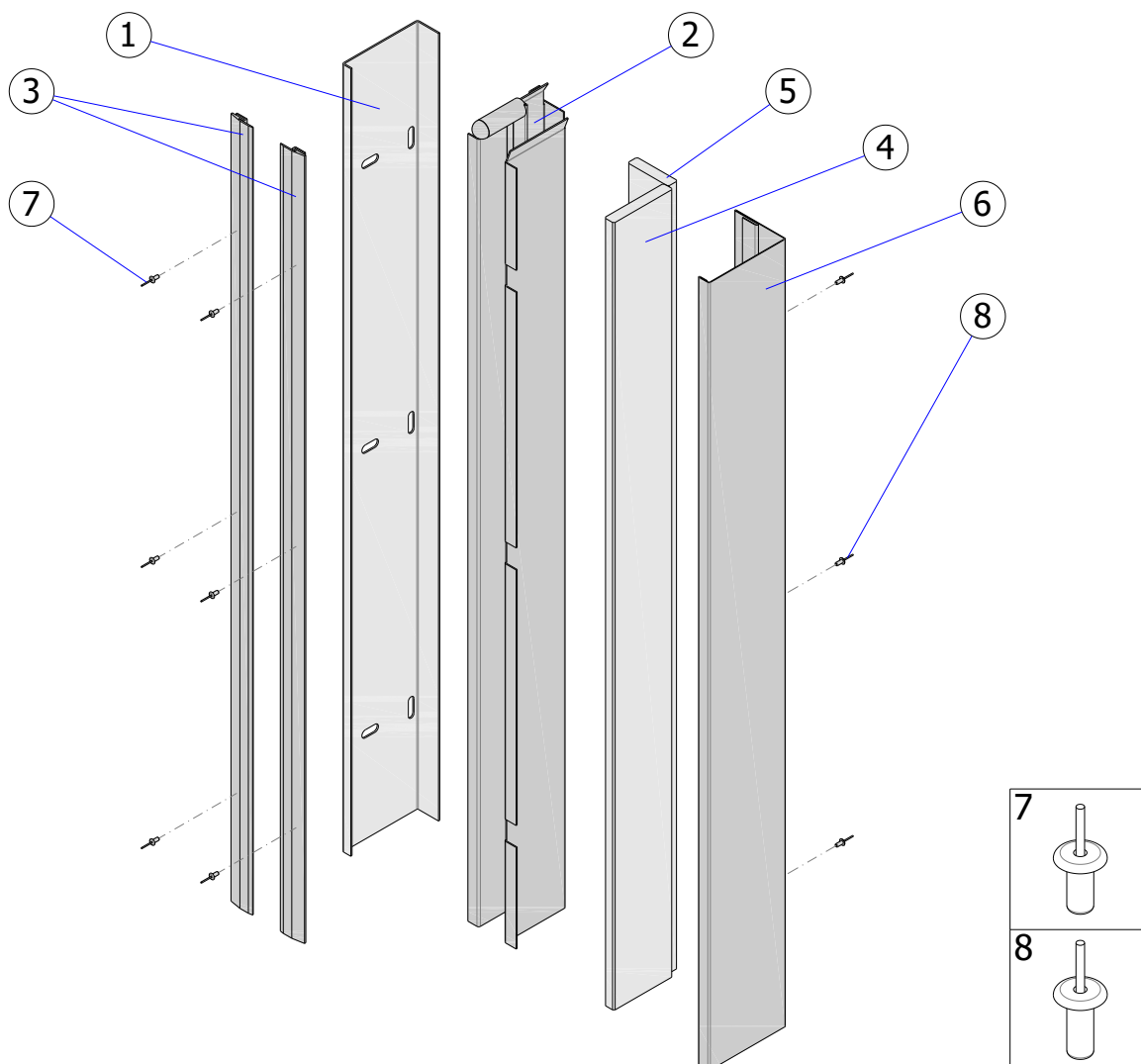
Rys. 21 – ISOiK-Ok30-01.21 [Prowadnica – wersja naścienna]
