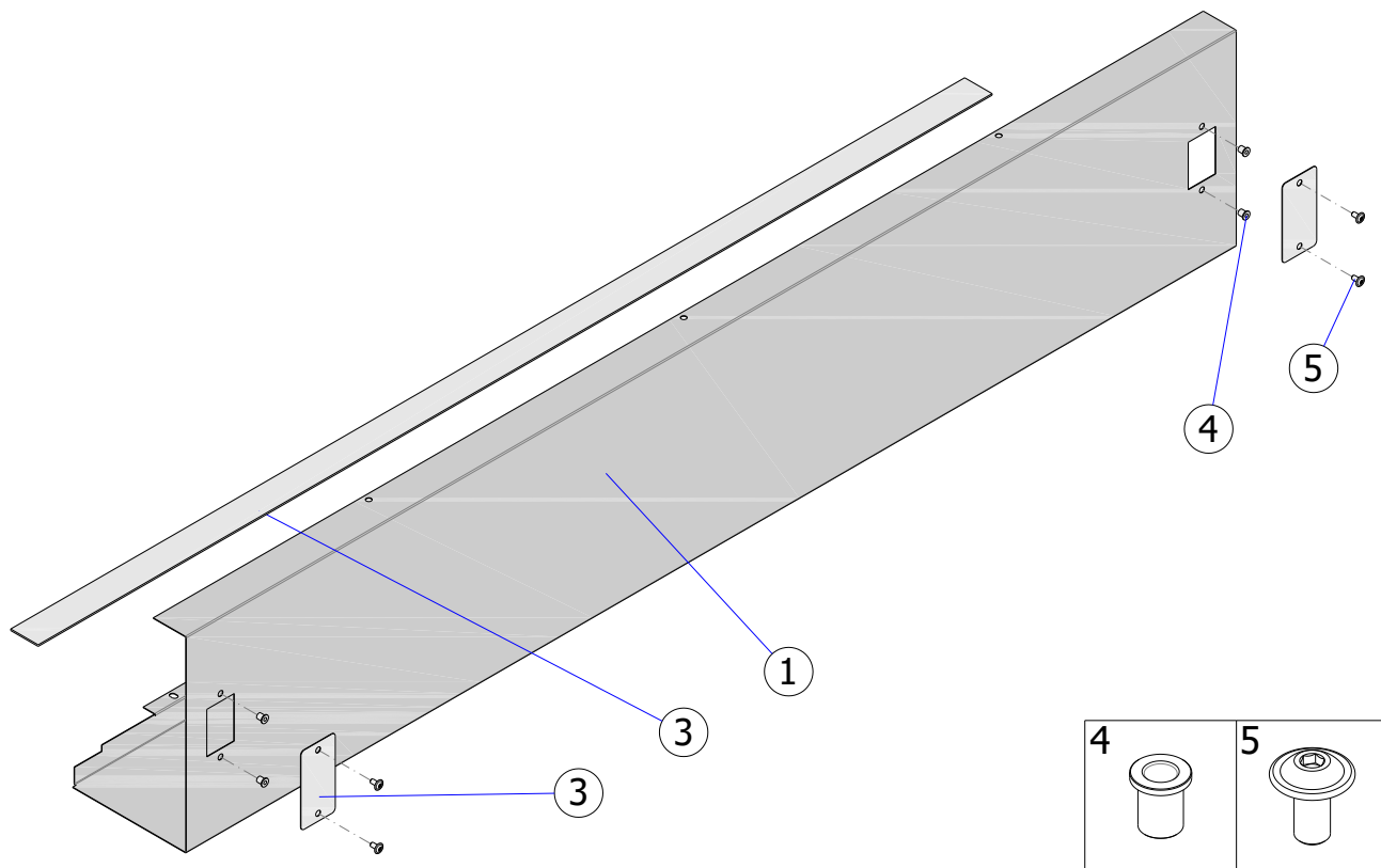
Rys. 28 – ISOiK-Ok30-01.28 [Osłona czołowa]
