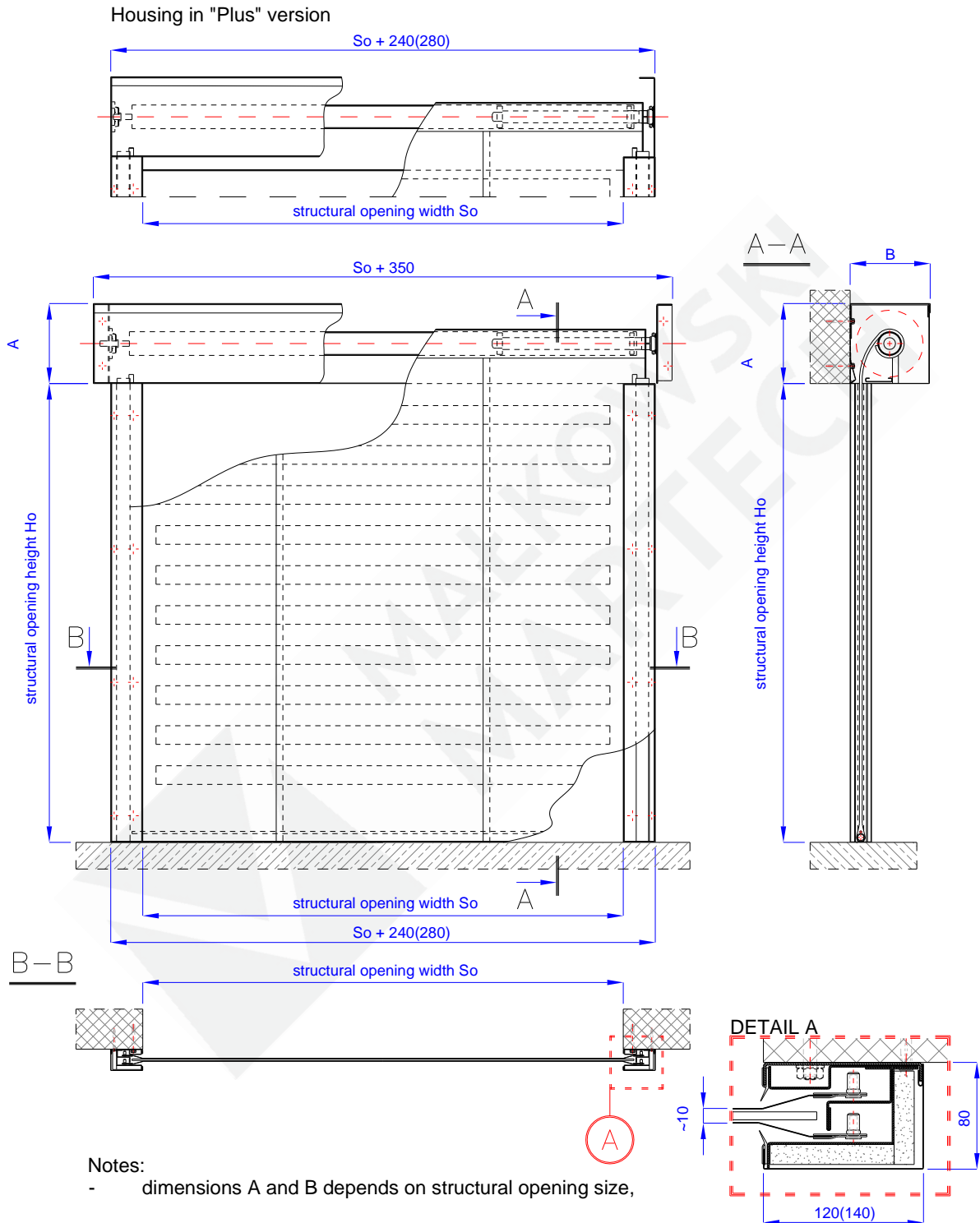
Fig. 1 – Fire protection curtain door MARC-Ok EI60
